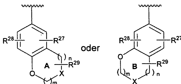
Chemische Formel 6:
