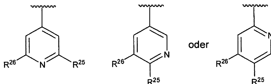
Chemische Formel 5:
