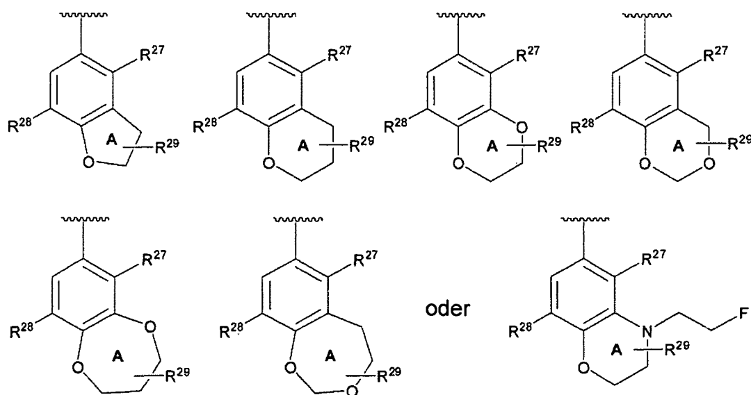
Chemische Formel 7:
