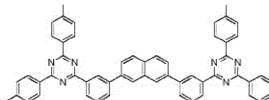
Composé 1-a-16
