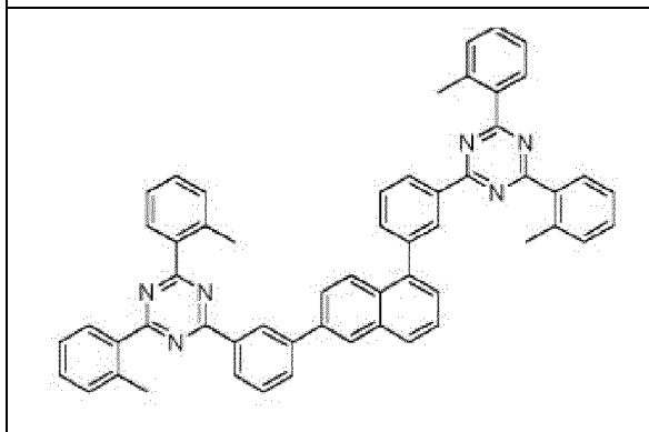
Composé 2-c-1
