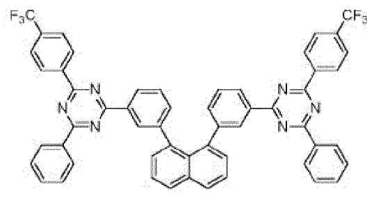
Composé 1-b-16
