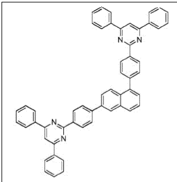
Composé 2-c-7
