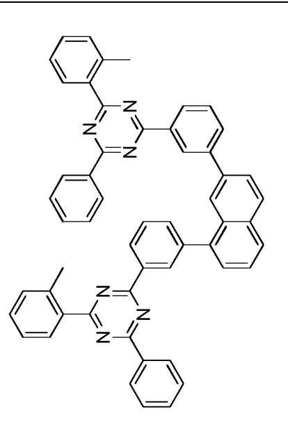
Verbindung 1-d-11
