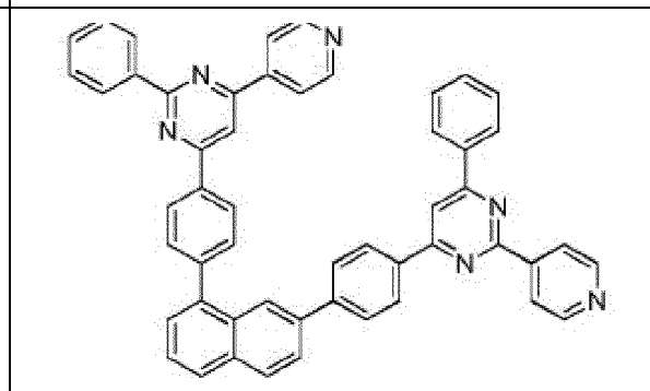
Composé 2-d-6
