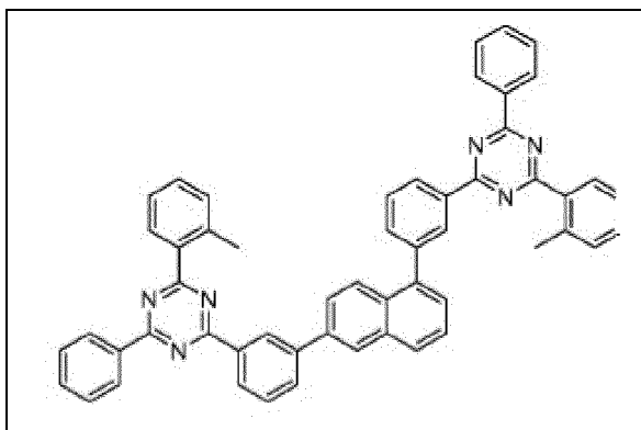
Composé 1-c-13
