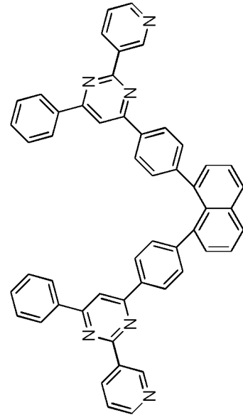
Verbindung 2-b-3
