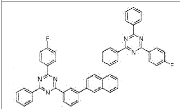
Composé 1-c-15
