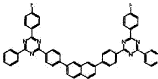
Composé 1-a-7
