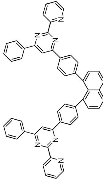
Verbindung 2-b-2
