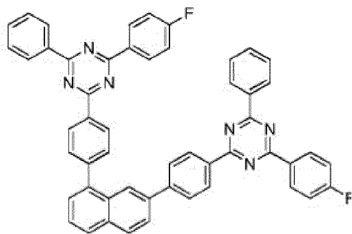
Composé 1-d-7
