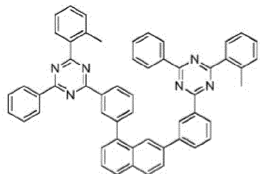
Composé 1-d-11
