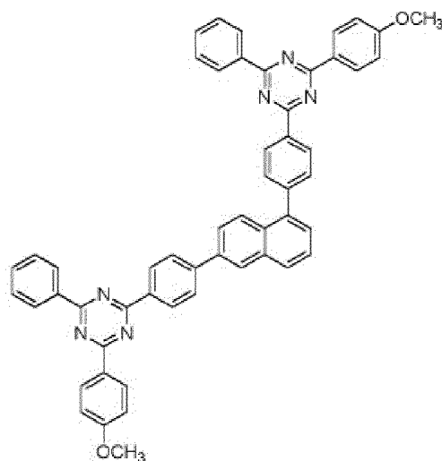
Composé 1-c-4
