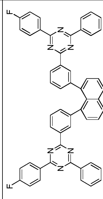
Verbindung 1-b-13
