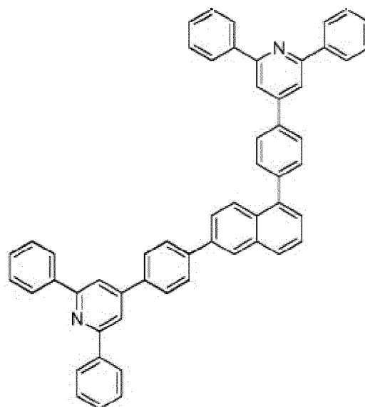
Composé 2-c-8
