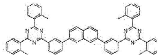
Composé 1-a-15
