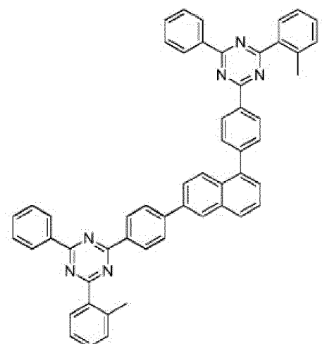
Composé 1-c-3
