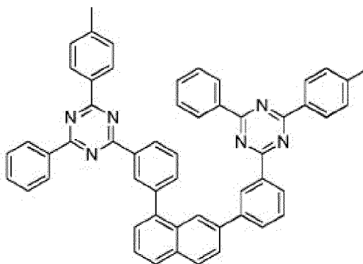
Composé 1-d-14
