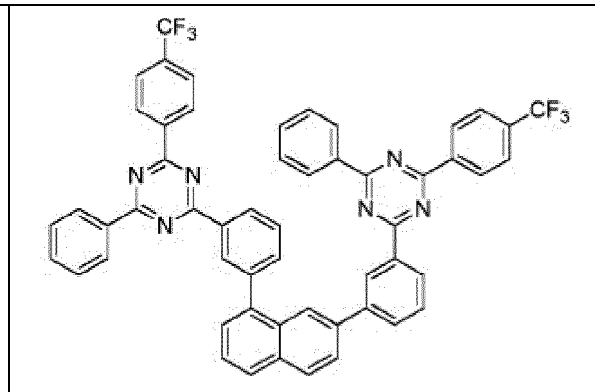
Composé 1-d-16
