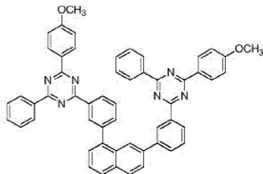
Composé 1-d-12
