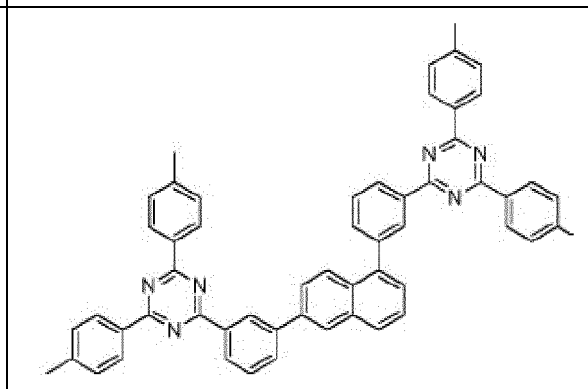
Composé 2-c-2
