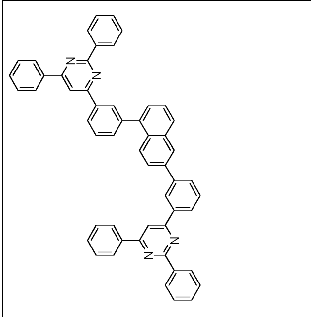
Verbindung 2-c-10
