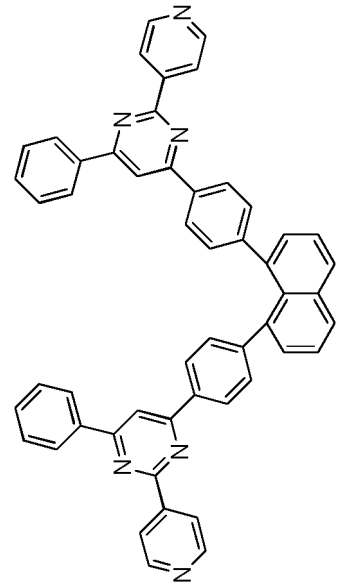
Verbindung 2-b-4
