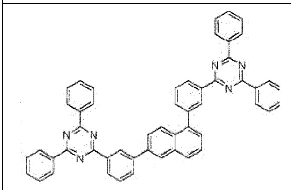
Composé 1-c-11
