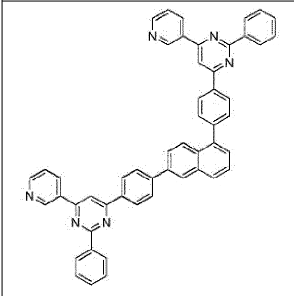
Composé 2-c-5
