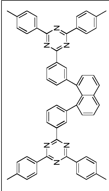
Verbindung 2-b-2
