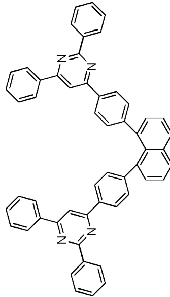
Verbindung 2-b-1
