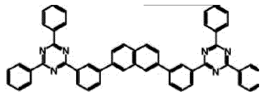
Composé 1-a-7
