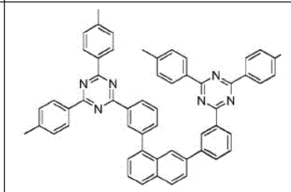
Composé 2-d-2
