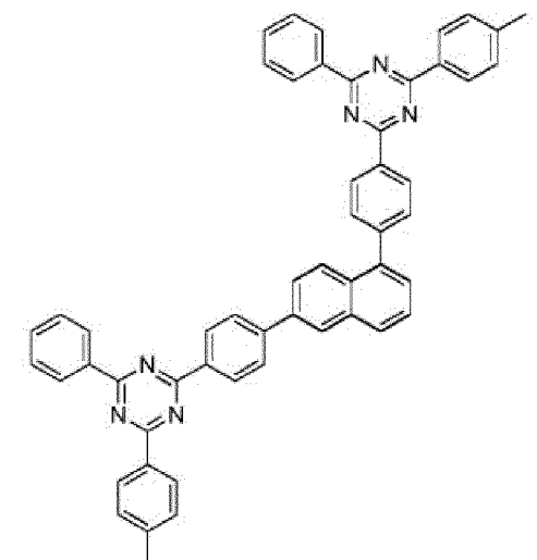
Composé 1-c-6
