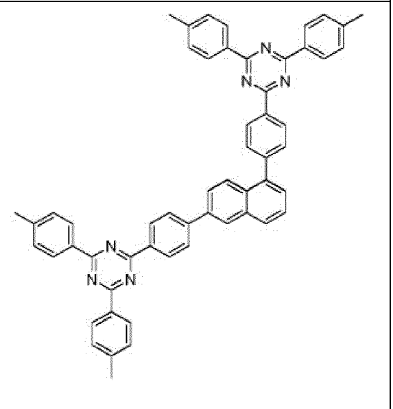
Composé 1-c-10
