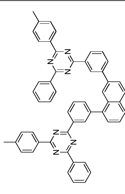
Verbindung 1-d-12
