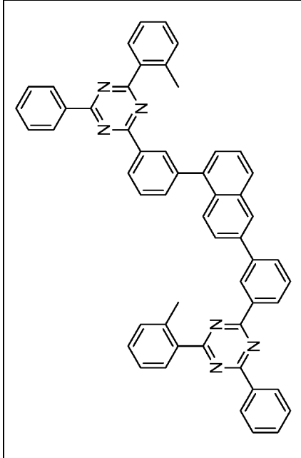
Verbindung 1-c-13
