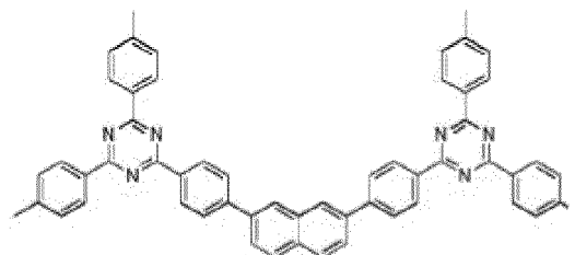
Composé 1-a-15
