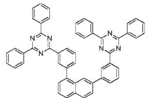
Composé 1-d-11
