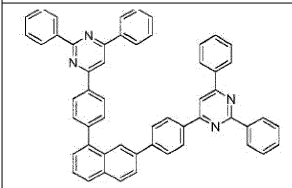
Composé 2-d-3
