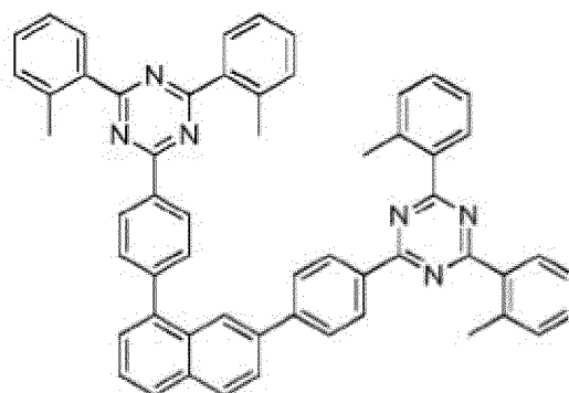
Composé 1-d-9
