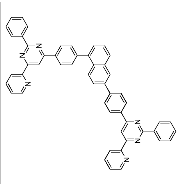
Verbindung 2-c-2
