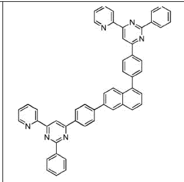
Composé 2-c-4
