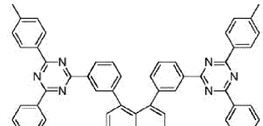
Composé 1-b-12
