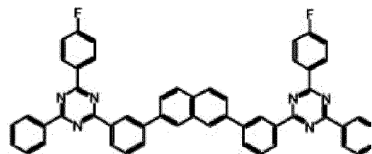
Composé 1-a-13
