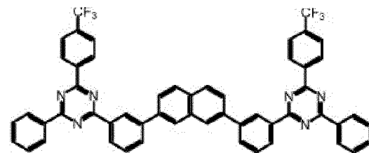
Composé 1-a-14
