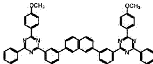
Composé 1-a-10
