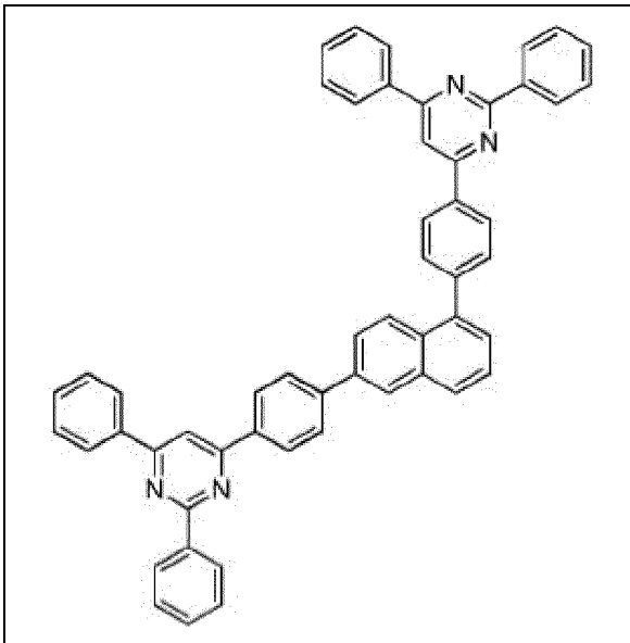
Composé 2-c-3
