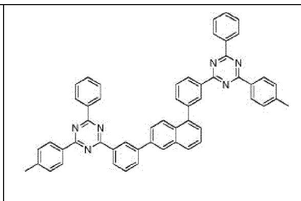
Composé 1-c-14
