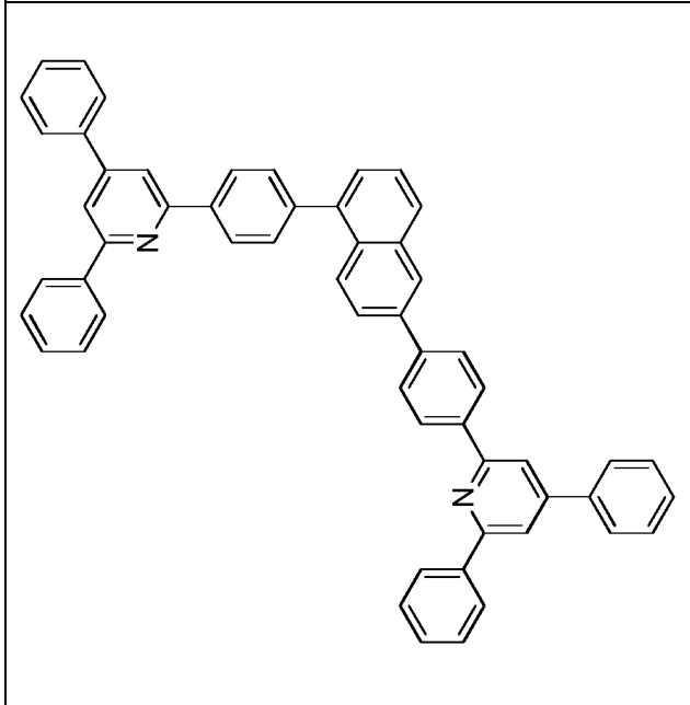
Verbindung 2-c-9
