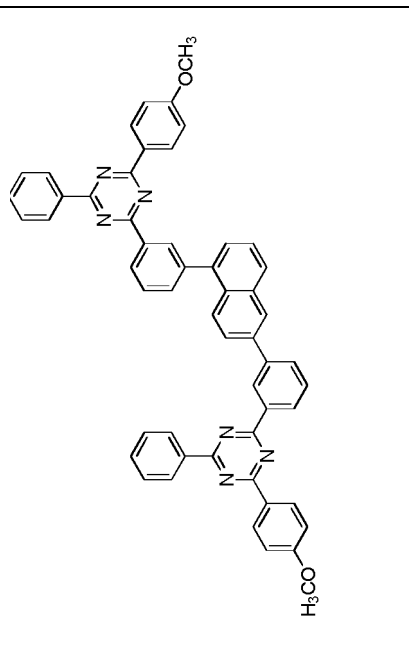
Verbindung 1-c-12
