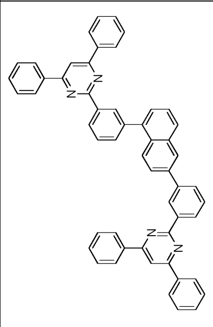
Verbindung 2-c-9
