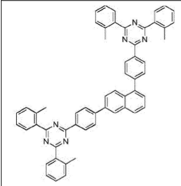
Composé 1-c-9
