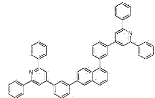
Composé 2-c-10
