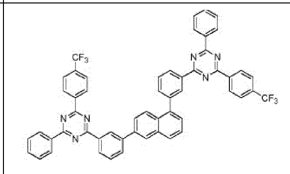
Composé 1-c-16
