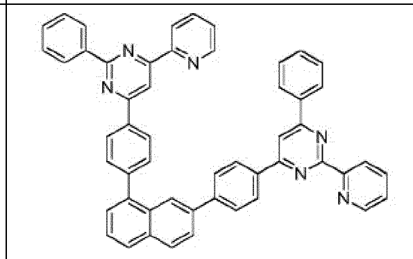
Composé 2-d-4
