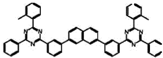
Composé 1-a-9
