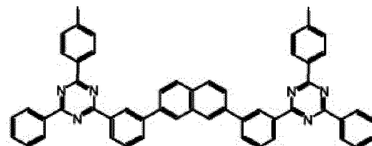
Composé 1-a-12
