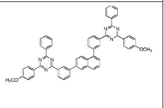
Composé 1-c-12
