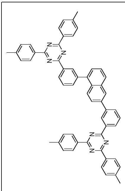
Verbindung 2-c-2
