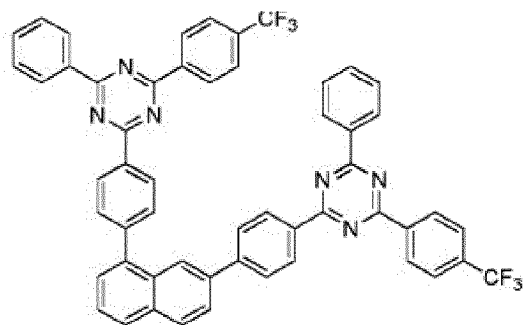
Composé 1-d-8
