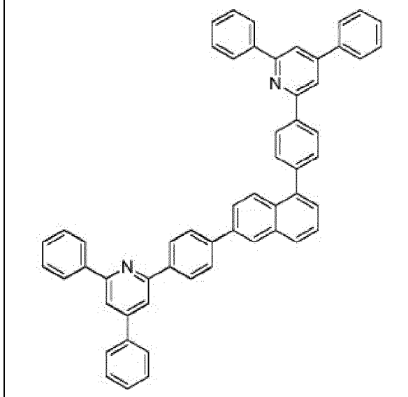
Composé 2-c-9
