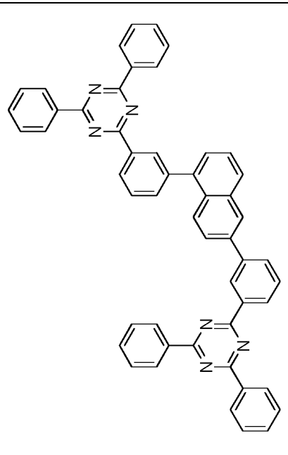
Verbindung 1-c-11
