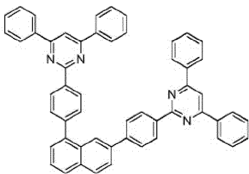
Composé 2-d-7
