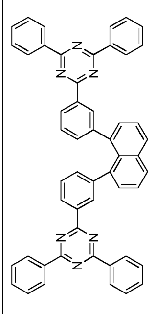
Verbindung 1-b-11
