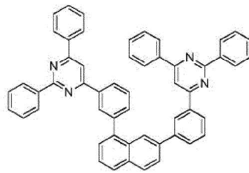
Composé 2-d-10
