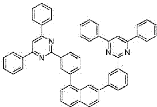
Composé 2-d-11
