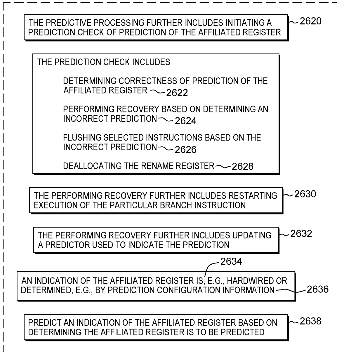
FIG. 26B
