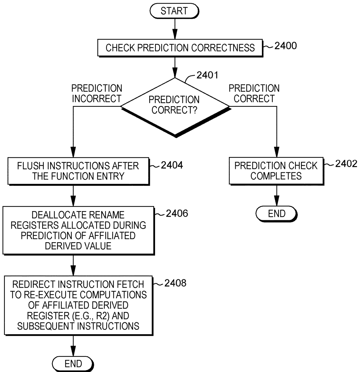
FIG. 24
