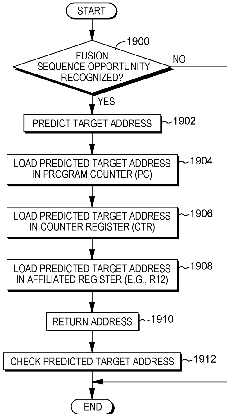
FIG. 19
