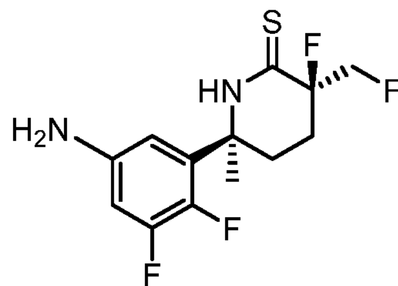
(3 R ,6 S )-6-(5-amino-2,3-difluorophenyl)-3-fluoro-3-(fluoromethyl)-6-methylpiperidine-2-thione
