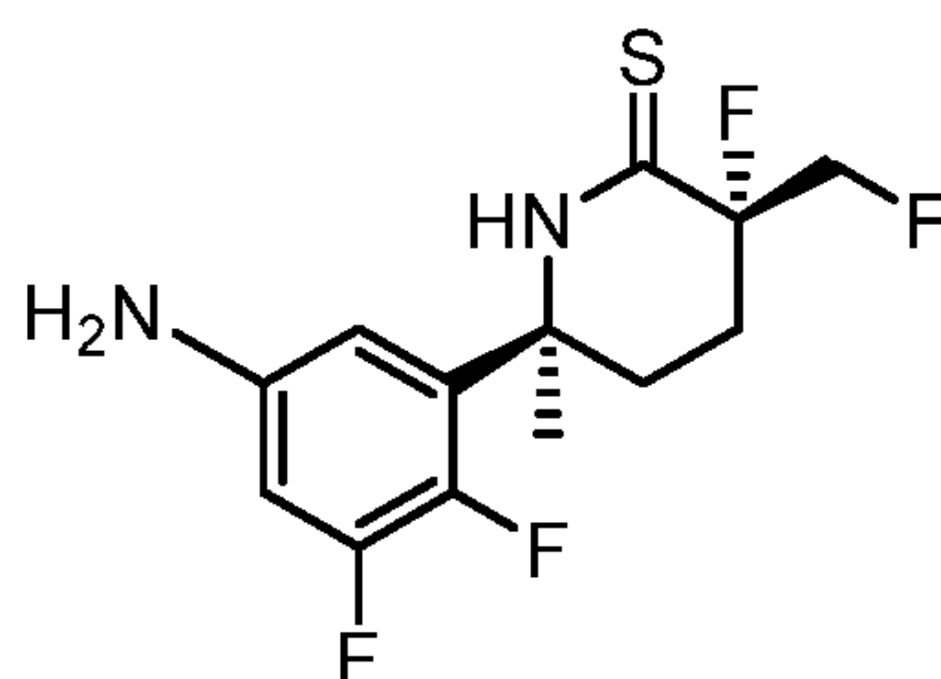
(3 S ,6 S )-6-(5-amino-2,3-difluorophenyl)-3-fluoro-3-(fluoromethyl)-6-methylpiperidine-2-thione
