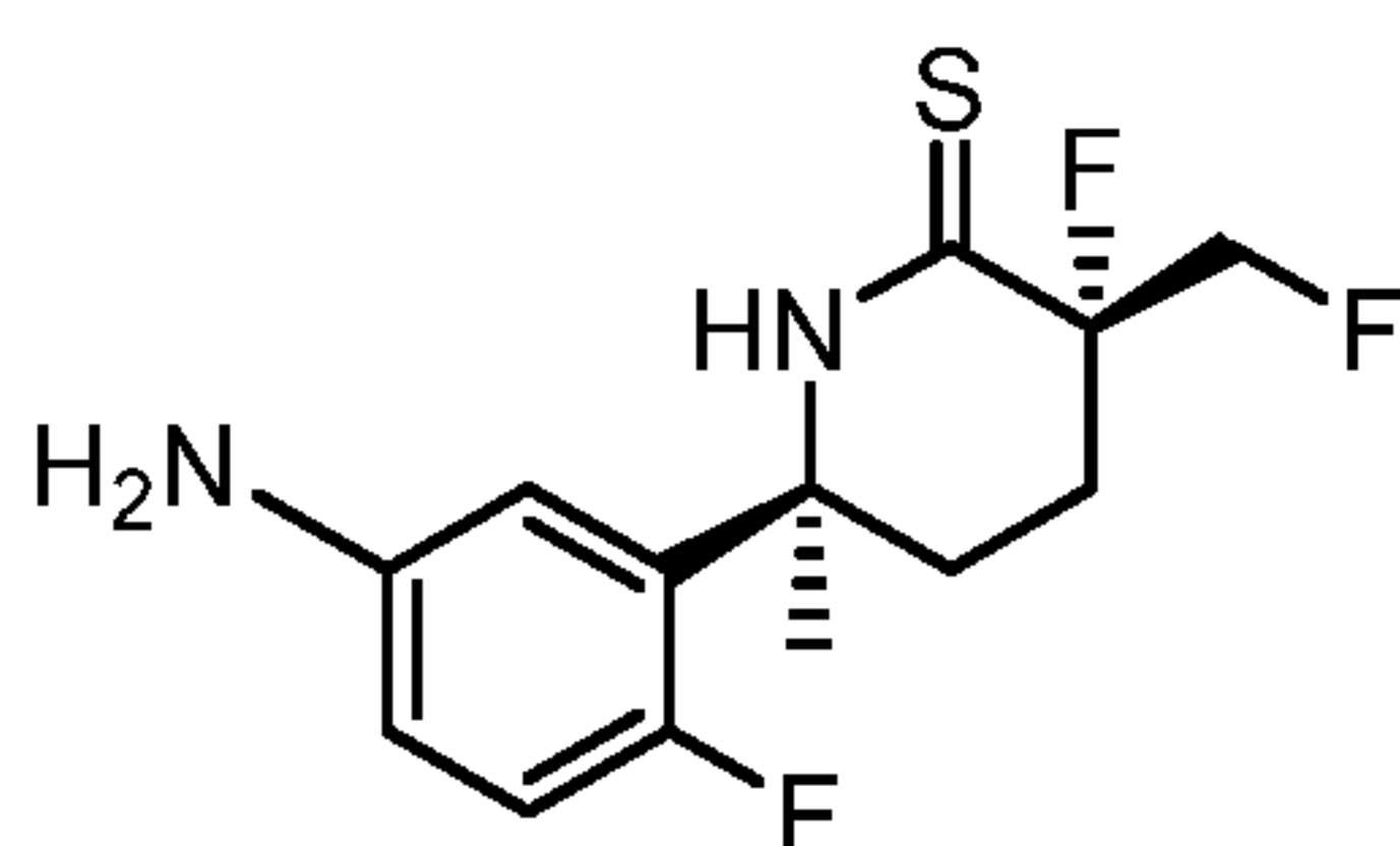
(3 S ,6 S )-6-(5-amino-2-fluorophenyl)-3-fluoro-3-(fluoromethyl)-6-methylpiperidine-2-thione
