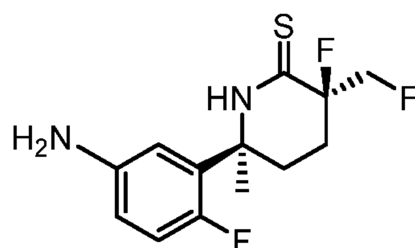
(3 R ,6 S )-6-(5-amino-2-fluorophenyl)-3-fluoro-3-(fluoromethyl)-6-methylpiperidine-2-thione
