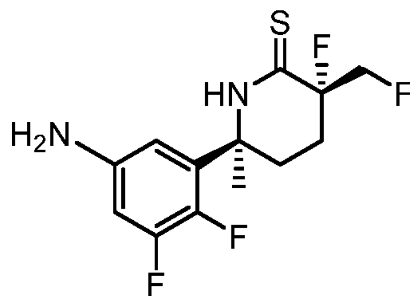
(3S,6S)-6-(5-amino-2,3-difluorophenyl)-3-fluoro-3-(fluoromethyl)-6-methylpiperidine-2-thione
