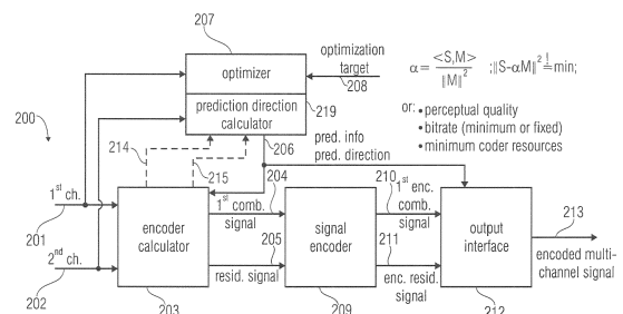
FIG 2 (AUDIO ENCODER)
