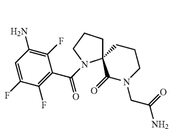
ST2828: SP32-Beta3-NH 2
