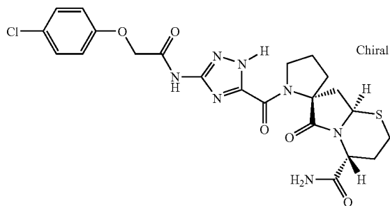
ST2941: PAM3-SP33-Beta8-NH 2
