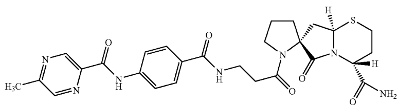
ST2826: PAM6-SP20-Beta8-NH 2
