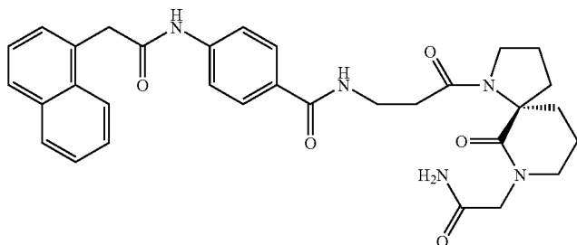
ST2793: PAM8-SP20-Beta3-NH 2
