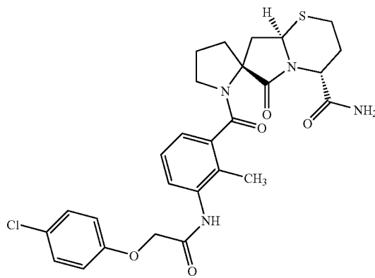
ST3375: PAM3-SP30-Beta8-NH 2
