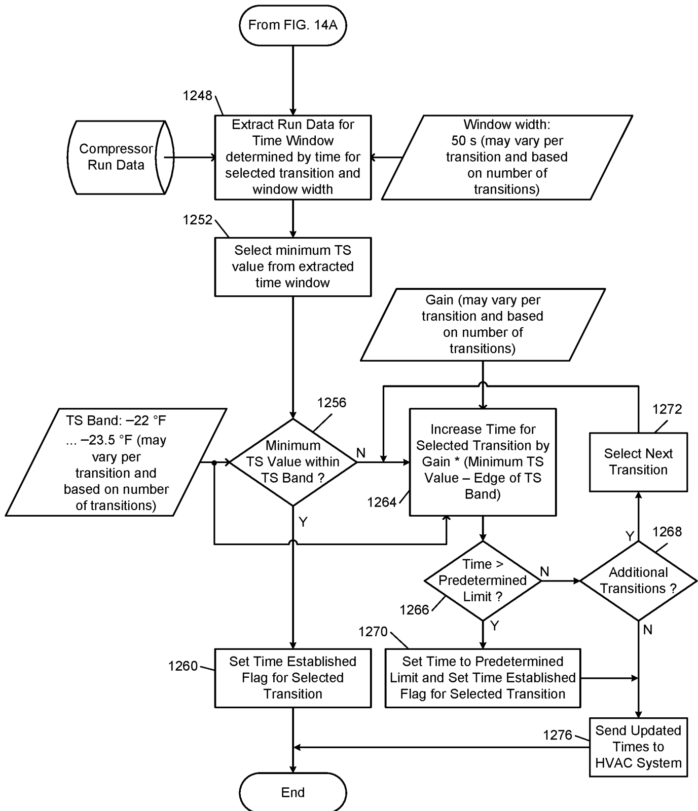
FIG. 14B
