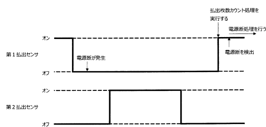
＜払出センサの作用図 パターンB＞
