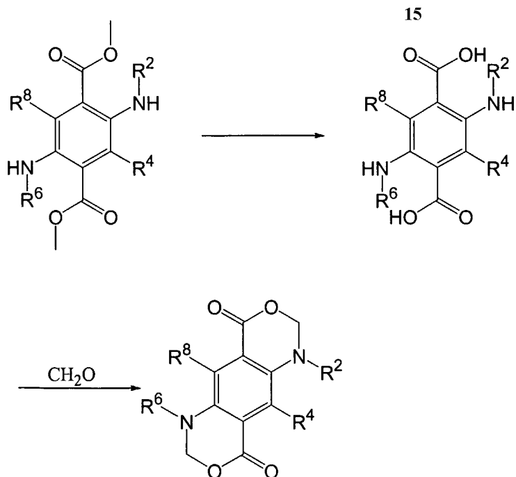
Formelschema II : Synthese der cyclisierten Verbindungen
