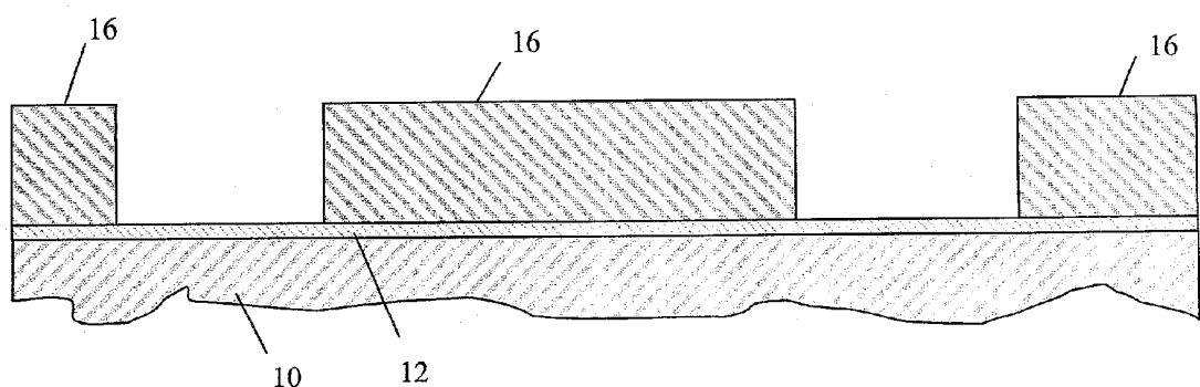
FIG. 9 (d) (PRIOR ART)
