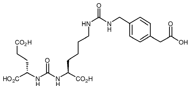
EC1170 (Exact Mass: 510.20 ; Mol. Wt.: 510.49)
