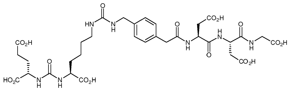
EC1168 (Exact Mass: 797.27 ; Mol. Wt.: 797.72)
