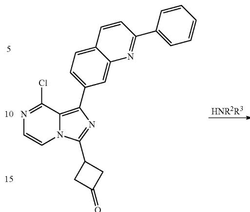
II-L1
