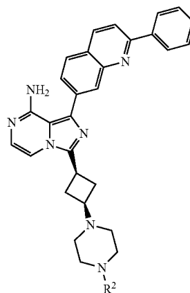
I-L1.2
