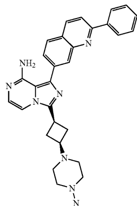
I-L1.1
