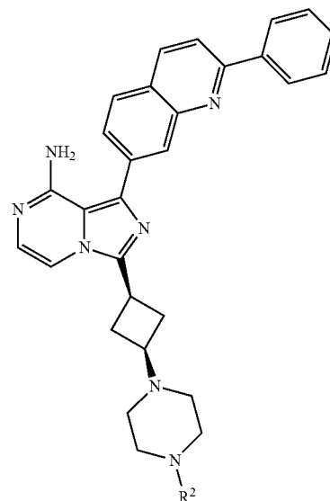
I-L1.2
