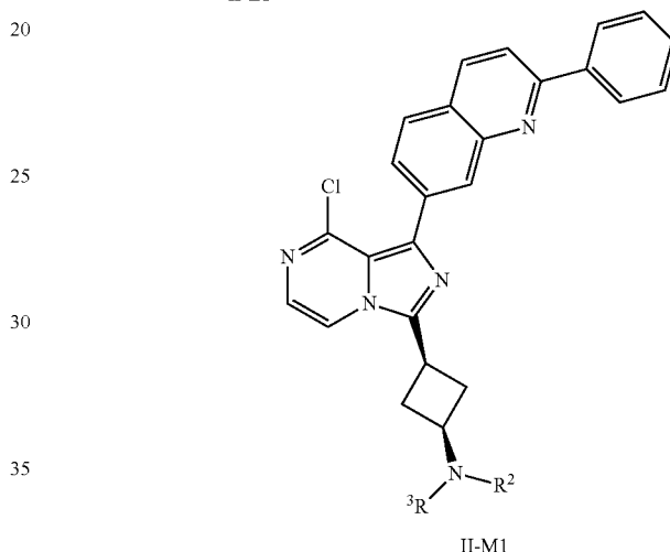
II-M1
