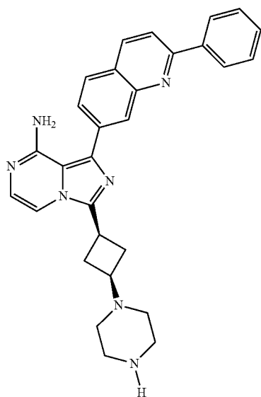
I-L1.1
