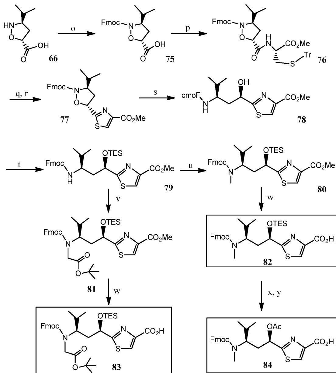
Figure 6. The synthesis of Tuv components of the antimitotic agents. Conditions: o): Fmoc-Cl, NaHCO 3 , THF/H 2 O, 95%; p): L-(S)-Tr-cysteine methyl ester, EDC, CH 2 Cl 2 , 87%; q): Ph 3 P=O, Tf 2 O, CH 2 Cl 2 ; r): MnO 2 , CH 2 Cl 2 , 76% (2 steps); s): Mo(CO) 6 , CH 3 CN/H 2 O, 87%; t): TES-Cl, Pyr., 95%; u): NaH, THF, CH 3 I, 90%; v): NaH, THF, BrCH 2 COOtBu, 0°C, 87%; w): HOSnMe 3 , ClCH 2 CH 2 Cl, 80°C; ~90%; x): Bu 4 NF, THF; y): Ac 2 O, Pyr. 81%.
