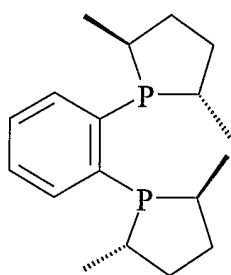
(S,S)-"Me-DuPhos",
