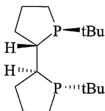
(S,S)-"Me-DuPhos",
