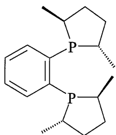
( S,S )-"Me-DuPhos",
