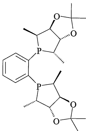
( S,S,S,S )-"Me-KetalPhos",
