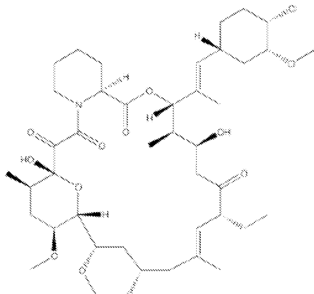
Pimecrolimus
