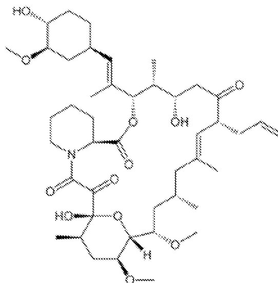
Tacrolimus
