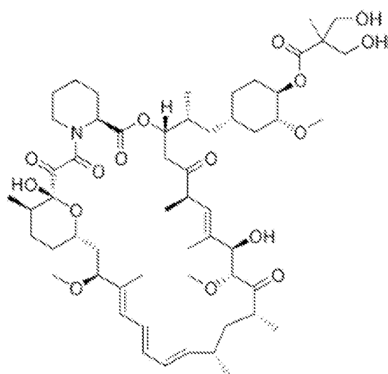
Temsirolimus
