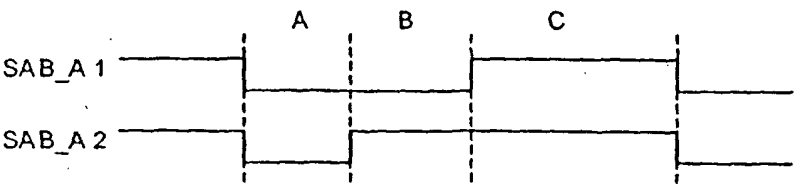
Figure 5 Micro con troller PWM ou tput
