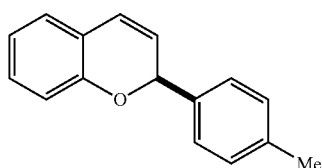
2e 73%, 93:7 er
