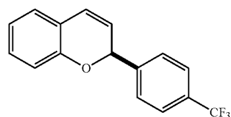
2j 81%, 83:17 er
