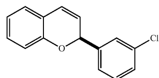
2i 81%, 93:7 er
