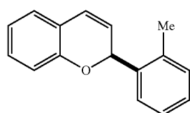
2d 72%, 92:8 er
