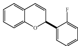
2g 75%, 91:9 er
