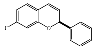
2m 69%, 90:10 er
