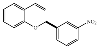
2l 71%, 92:8 er
