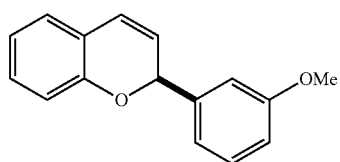
2f 78%, 94:6 er
