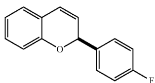
2h 84%, 95:5 er
