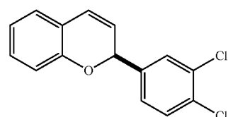
2k 74%, 90:10 er
