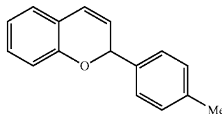
2-(p-Tolyl)-2H-chromene (2e)
