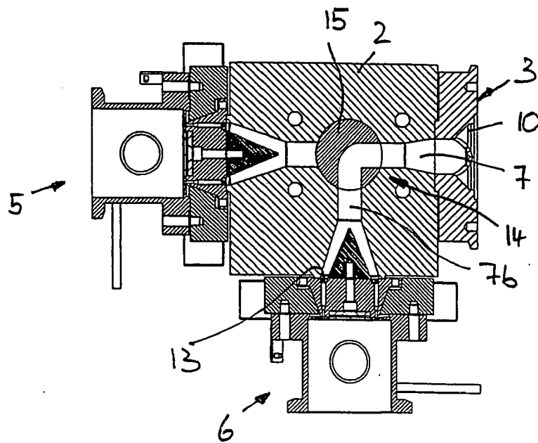
SCHNITTDARSTELLUNG C-C
