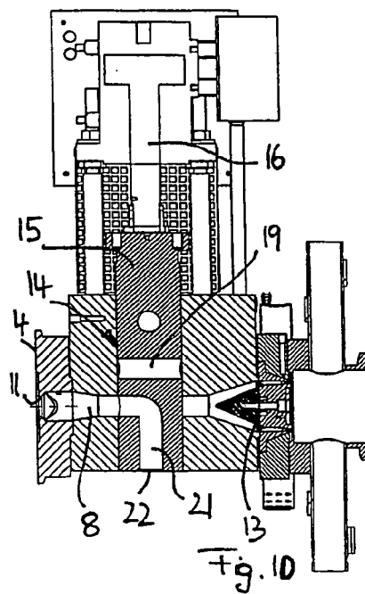
SCHNITTDARSTELLUNG C-C
