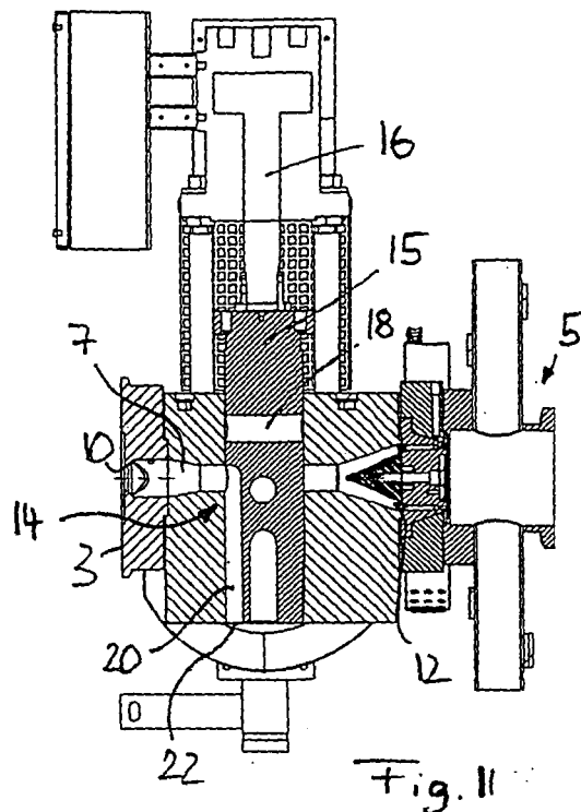
SCHNITTDARSTELLUNG D-D
