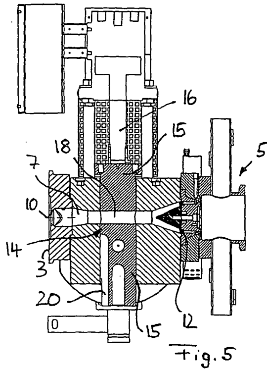
SCHNITTDARSTELLUNG D-D
