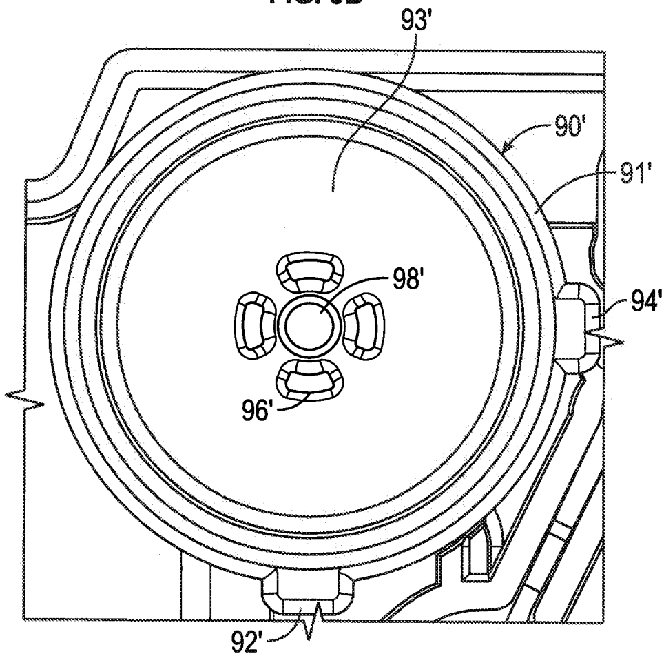
FIG. 8C
