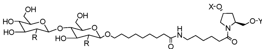
MONOMER 26
