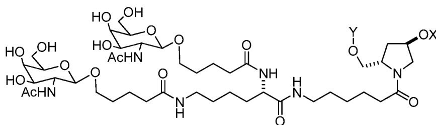
MONOMER 7
