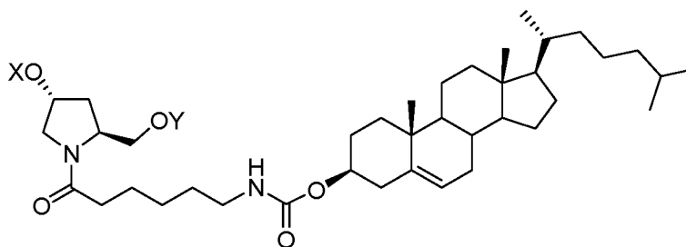
MONOMER 30.
