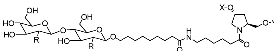
MONOMER 29
