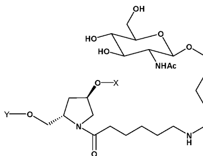
MONOMER 15.
