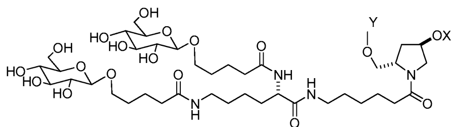
MONOMER 8
