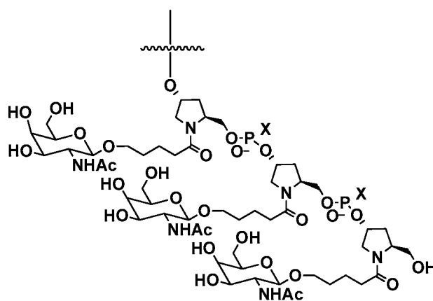
MONOMER 20
