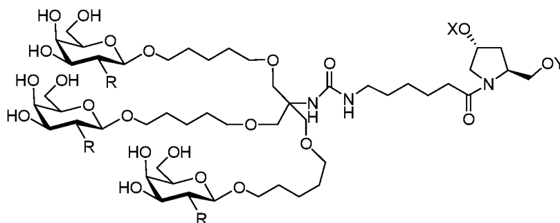
MONOMER 27
