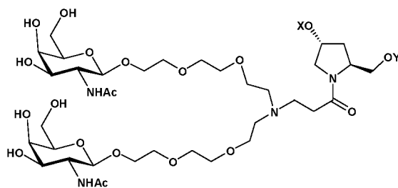
MONOMER 14.
