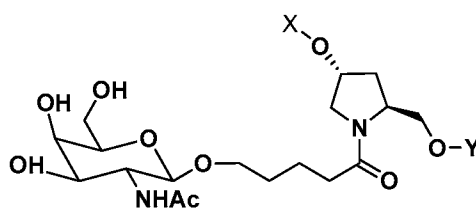
MONOMER 19.
