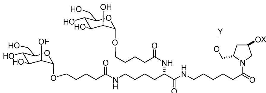
MONOMER 9
