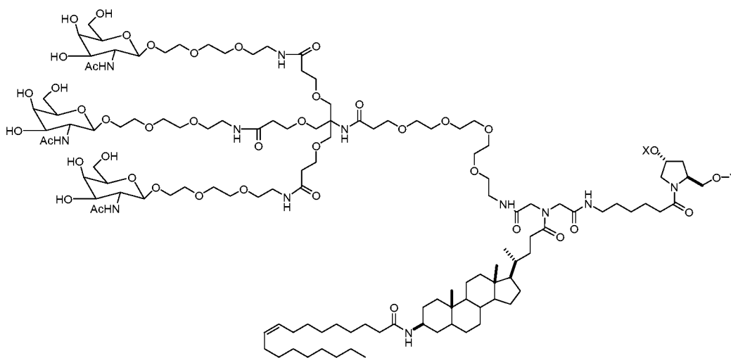
MONOMER 13.
