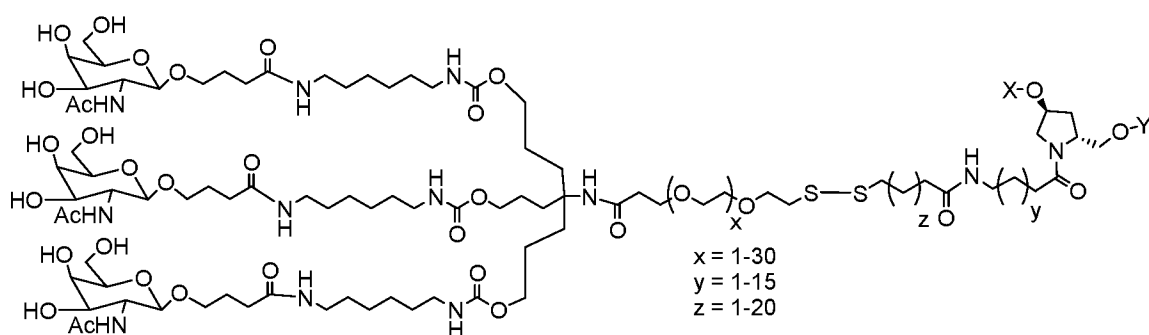
MONOMER 5
