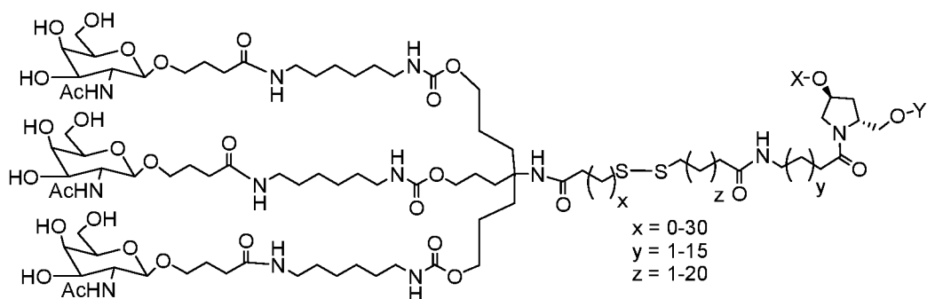
MONOMER 4
