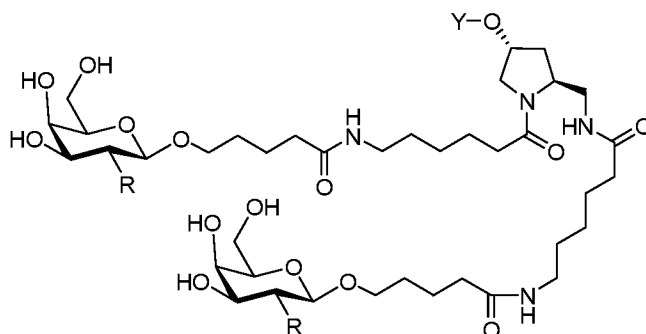
MONOMER 25.
