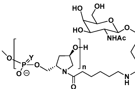
MONOMER 16
