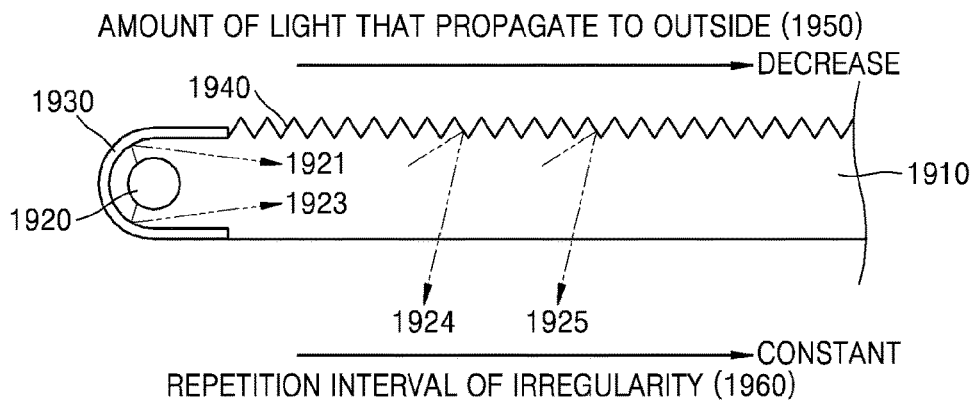
FIG. 19C
