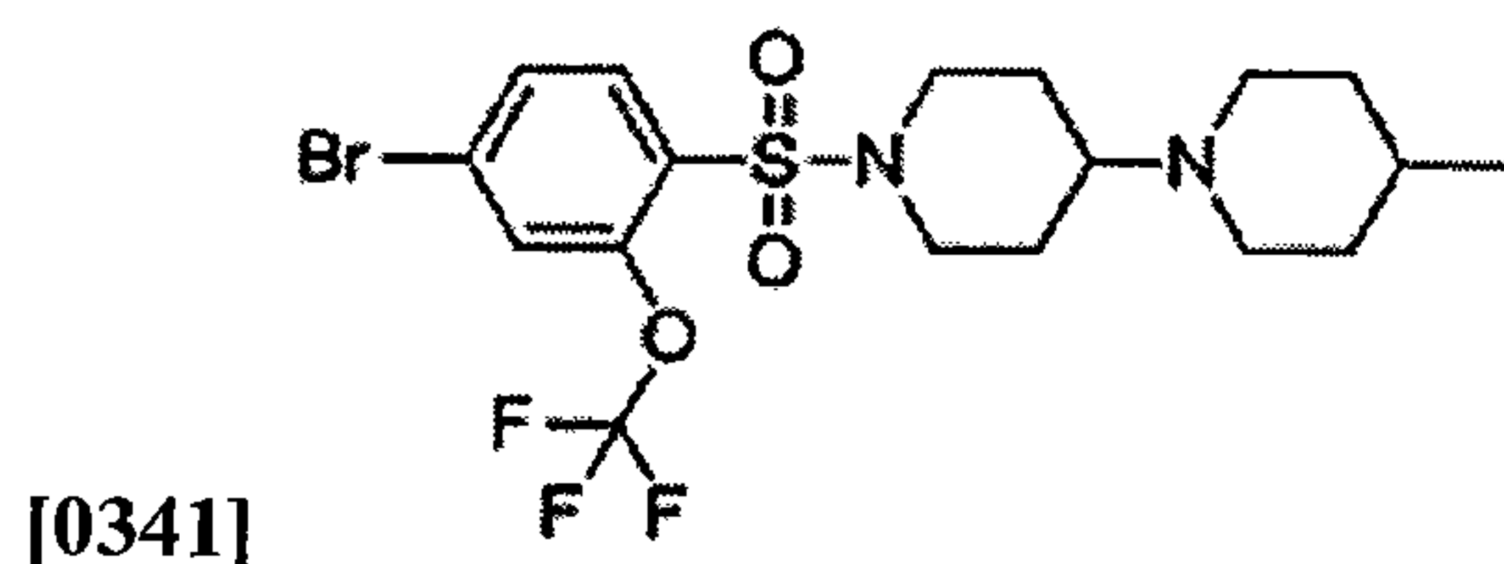
1'-((4-bromo-2-
