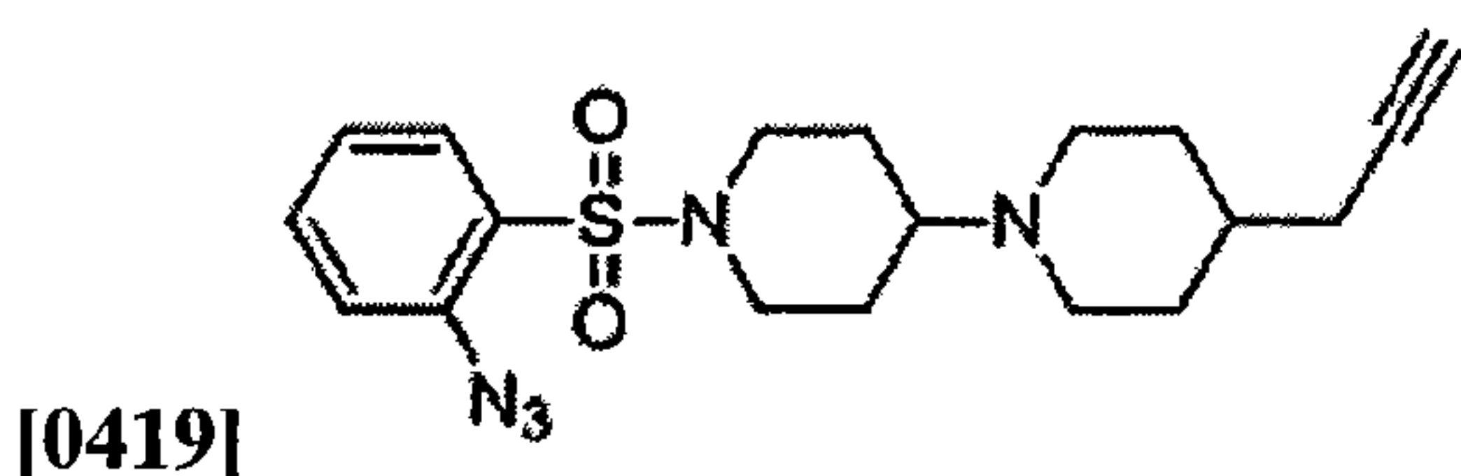
1'-((2-azidophenyl)sulfonyl)-4-(prop-2-yn-1-yl)-
