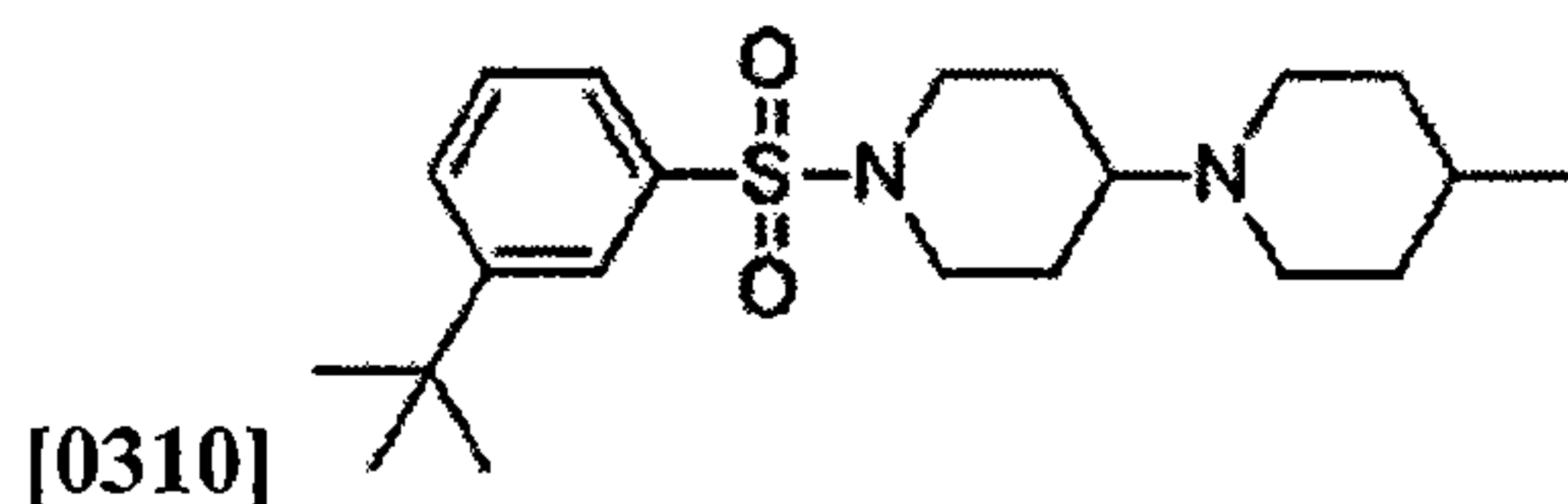
1'-((3-(tert-butyl)phenyl)sulfonyl)-4-methyl-1,4'-
