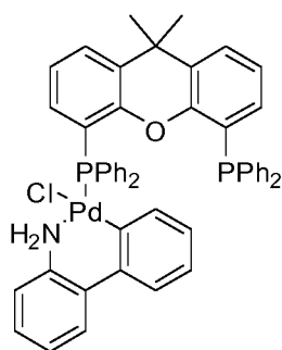
XantPhos-Pd-G2
