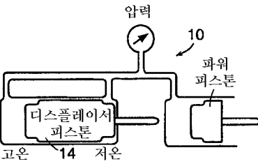
펌프 행정의 종료
