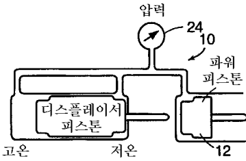
펌프 행정의 개시 준비
