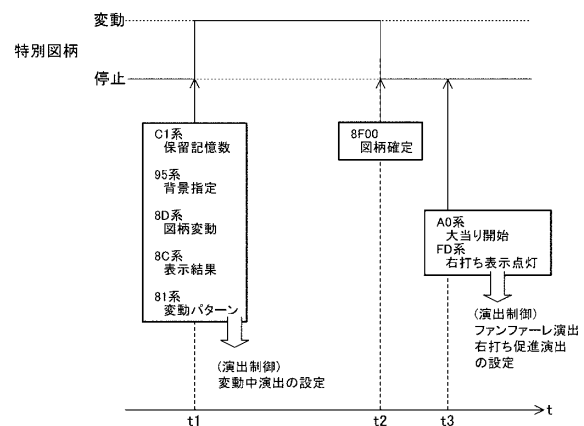
【図13-19】 当り変動中におけるタイミングチャート
