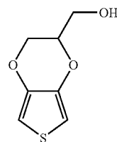
EDT-methanol
