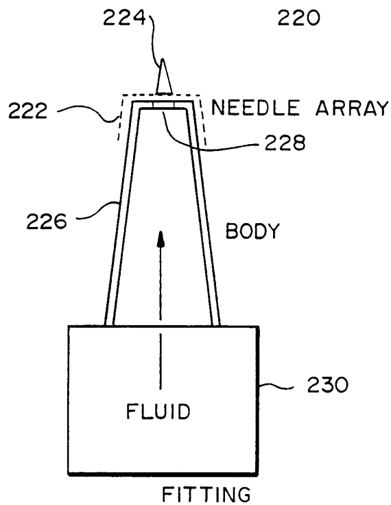
FIG. 11C
