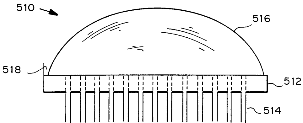
FIG. 20B
