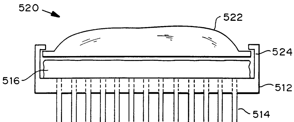
FIG. 20C
