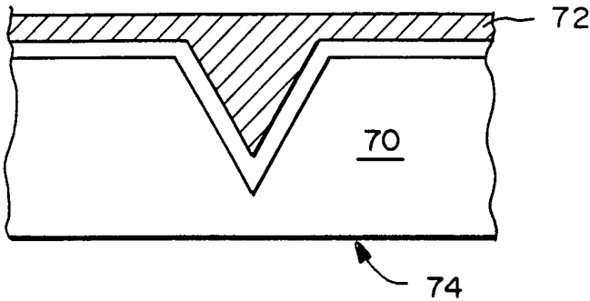
FIG. 8B
