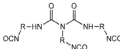
biuret trimer
