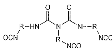
biuret trimer
