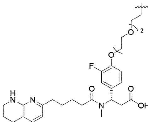
(Struktur 32a);
