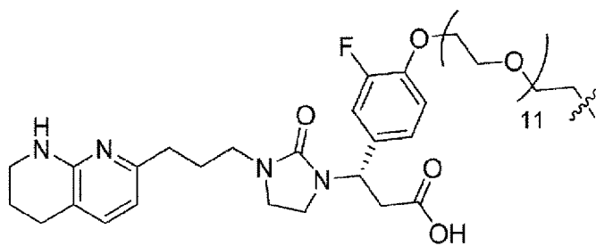
(Struktur 2.8a);
