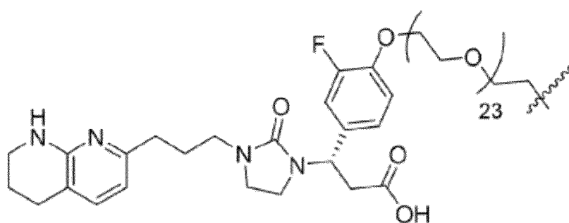
(Structure 2.9a) ;
