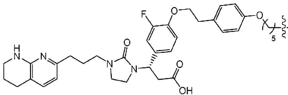
(Struktur 2.5a);
