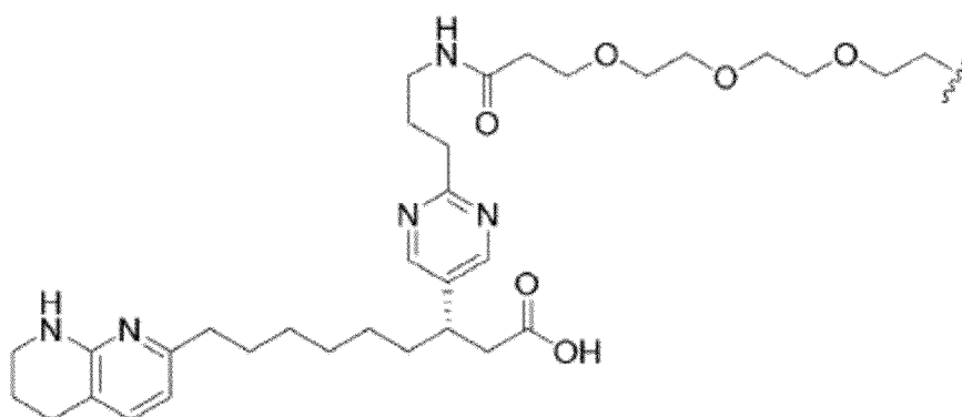
(Structure 39a) ;
