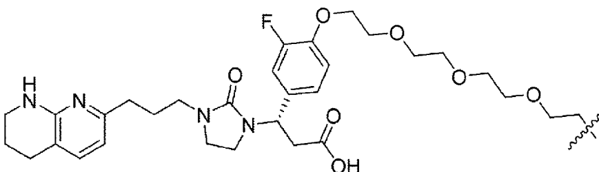
(Struktur 2a);
