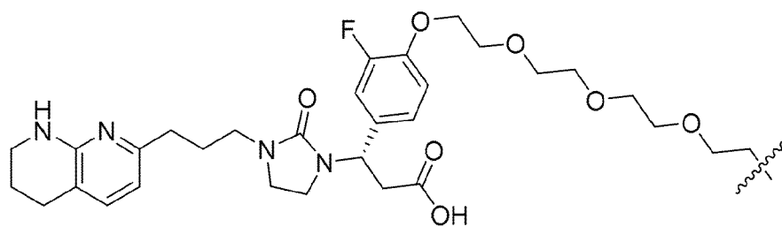
(Structure 2a);
