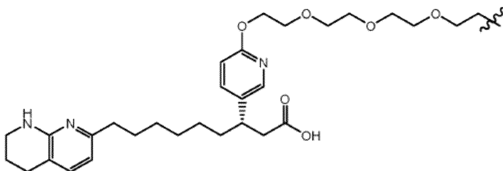
(Structure 29a) ;
