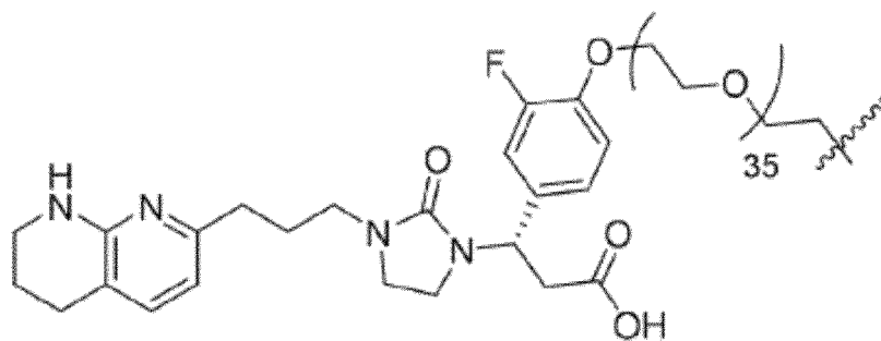
(Structure 2.10a) ;
