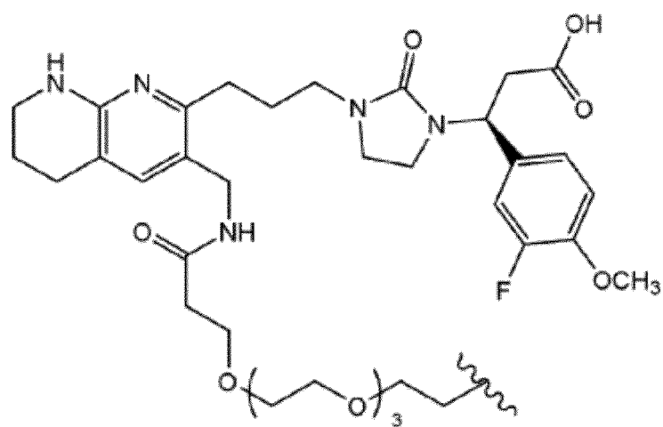
(Structure 2.5a) ;
