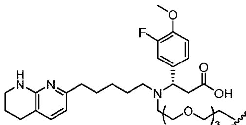
(Struktur 34a);
