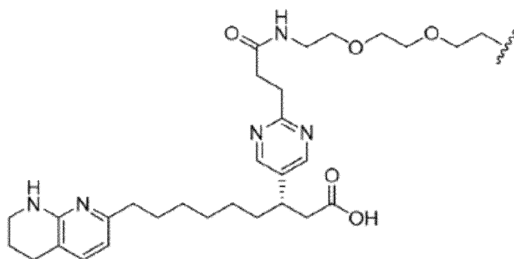
(Structure 38a) ;
