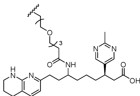
(Structure 40a).
