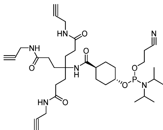
(Structure 400).
