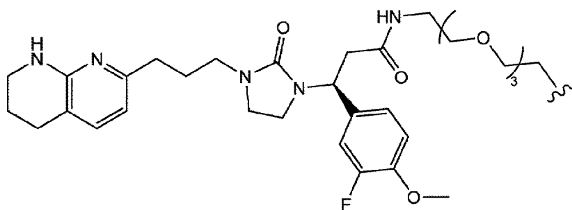
(Struktur 2.7a);
