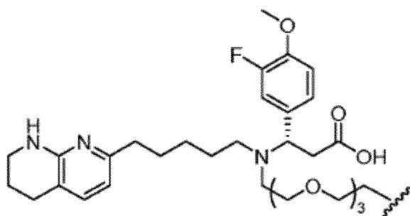
(Structure 34a) ;
