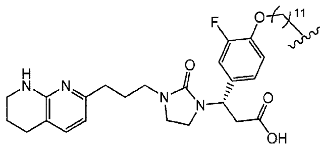
(Struktur 2.1a);
