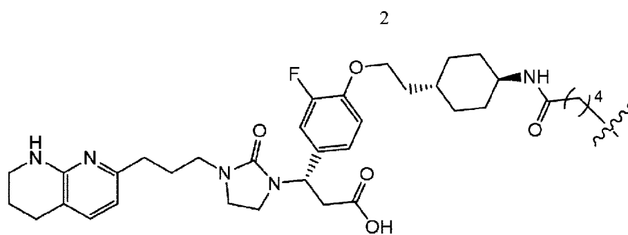
(Struktur 2.3a);
