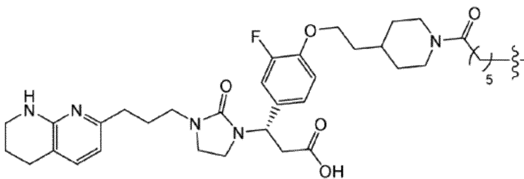
(Structure 2.2a) ;
