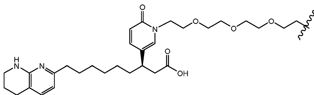
(Structure 31a);
