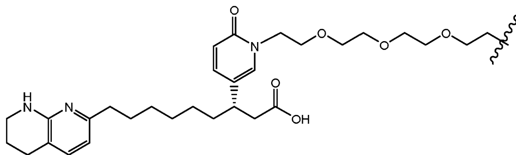
(Structure 30a);
