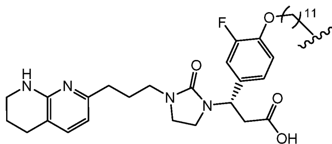
(Structure 2.1a).
