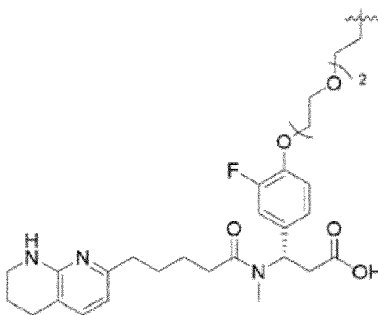
(Structure 32a) ;
