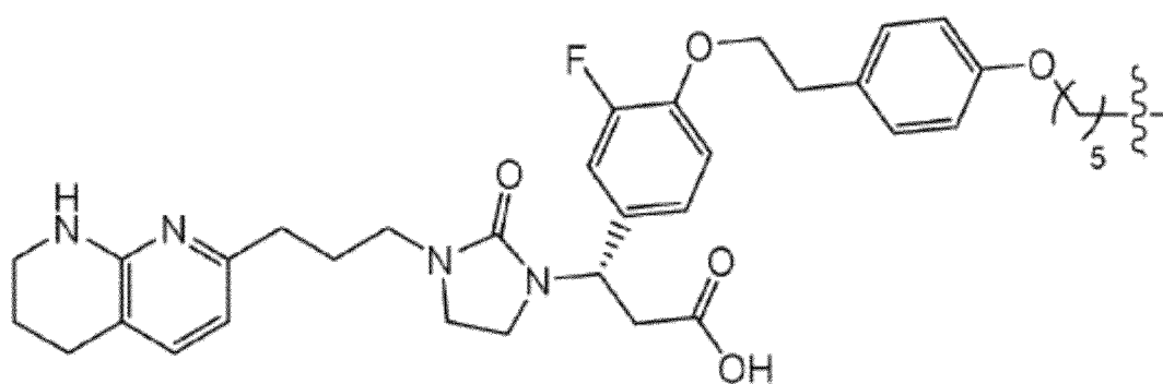
(Structure 2.5a) ;
