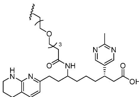
(Structure 41a).
