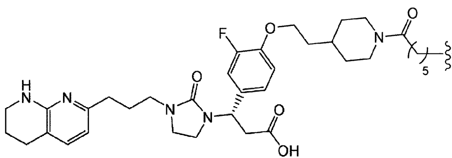
(Struktur 2.2a);
