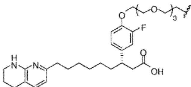
(Structure 36a) ;
