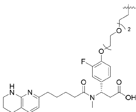
(Structure 32a);
