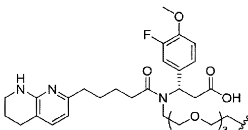
(Struktur 33a);
