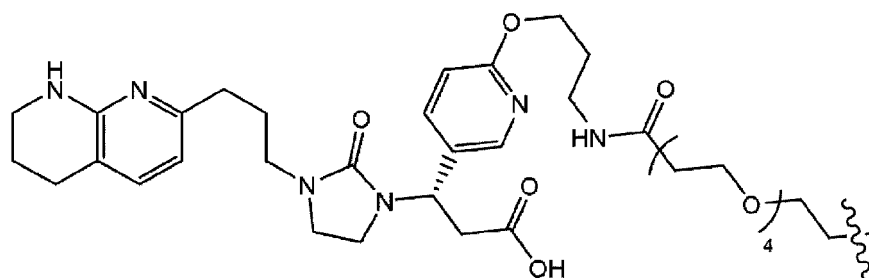
(Struktur 1a);
