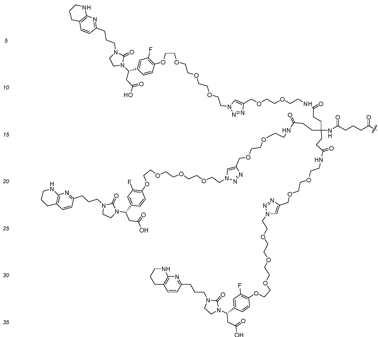
(Structure 700)
