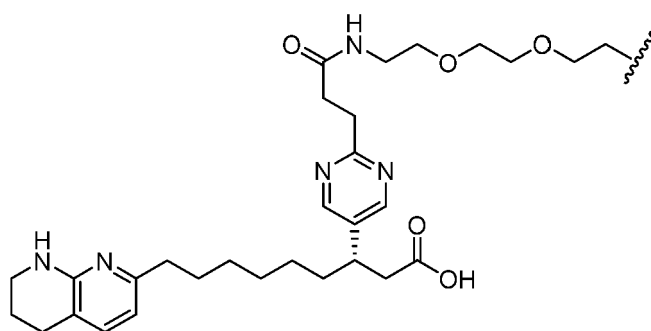
(Structure 38a);
