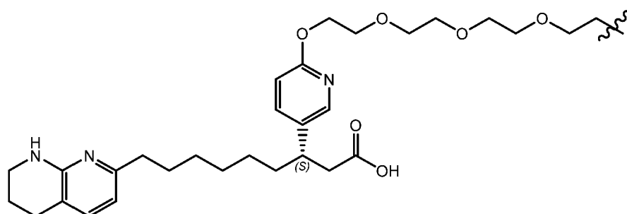
(Structure 29a).
