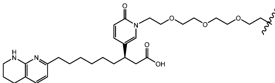
(Structure 31a);
