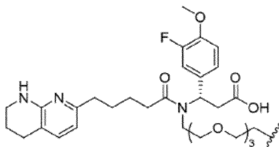
(Structure 33a) ;
