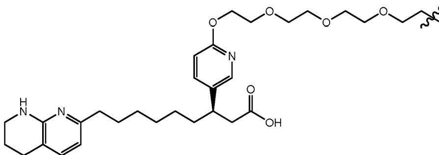
(Structure 28a);
