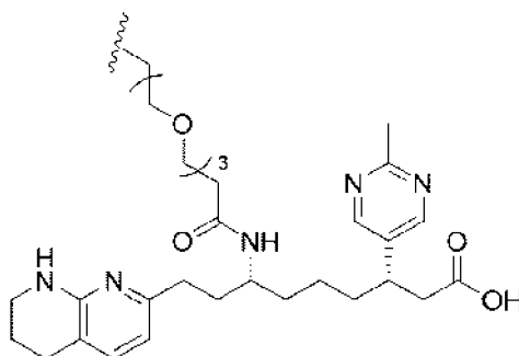
(Structure 41a)
