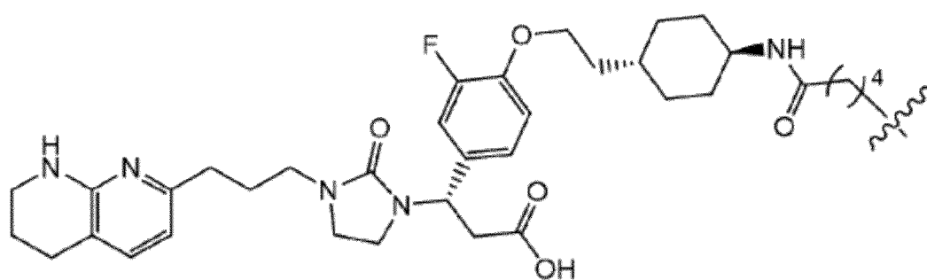
(Structure 2.3a) ;
