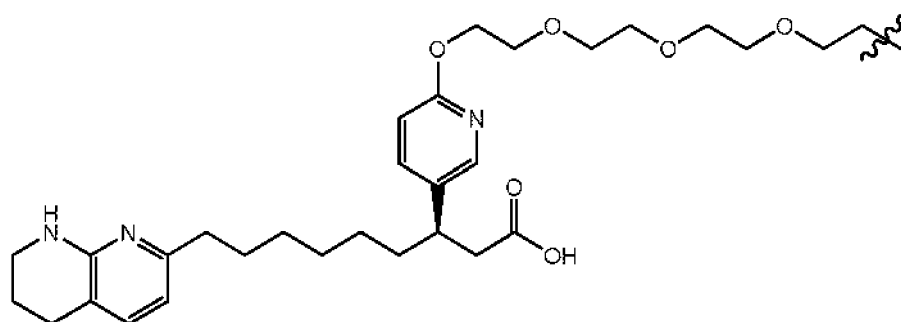
(Structure 28a) ;
