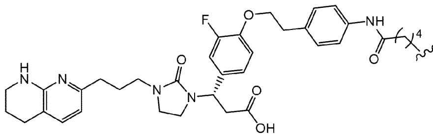
(Structure 2.4a);
