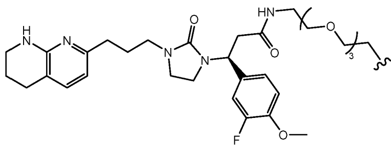
(Structure 2.7a);
