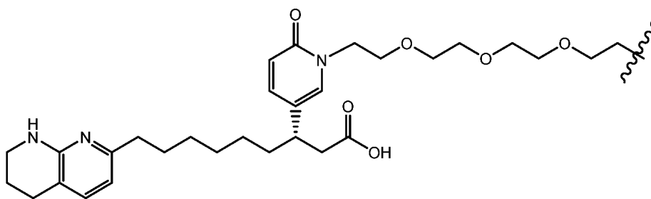
(Structure 30a);
