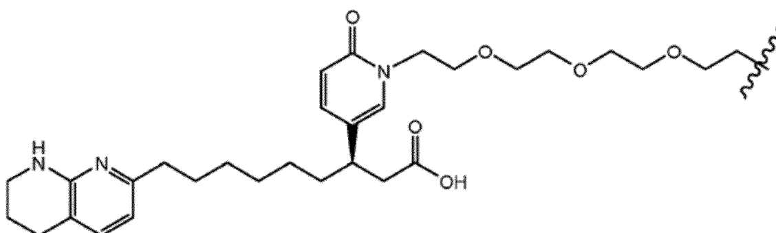
(Structure 31a) ;
