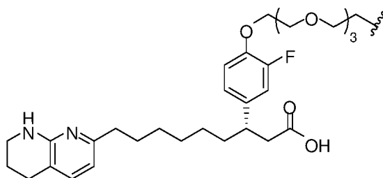
(Structure 36a);
