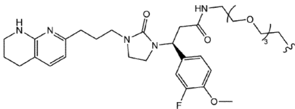
(Structure 2.6a) ;
