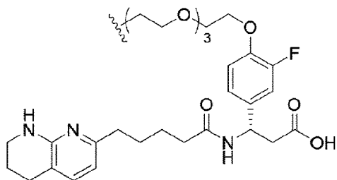
(Struktur 37a);
