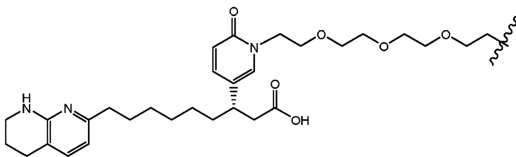
(Struktur 30a);
