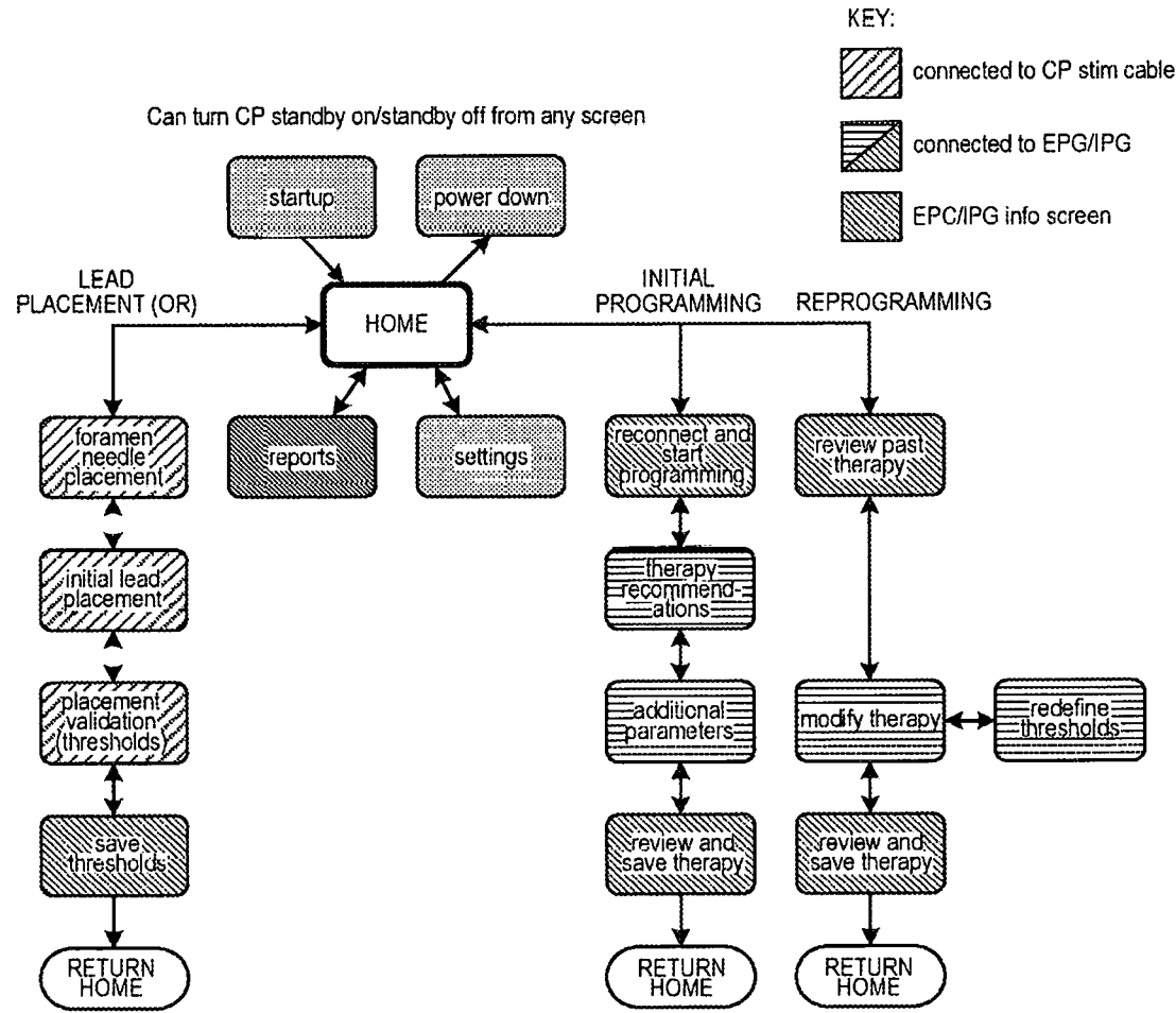
CP GUI Workflow
