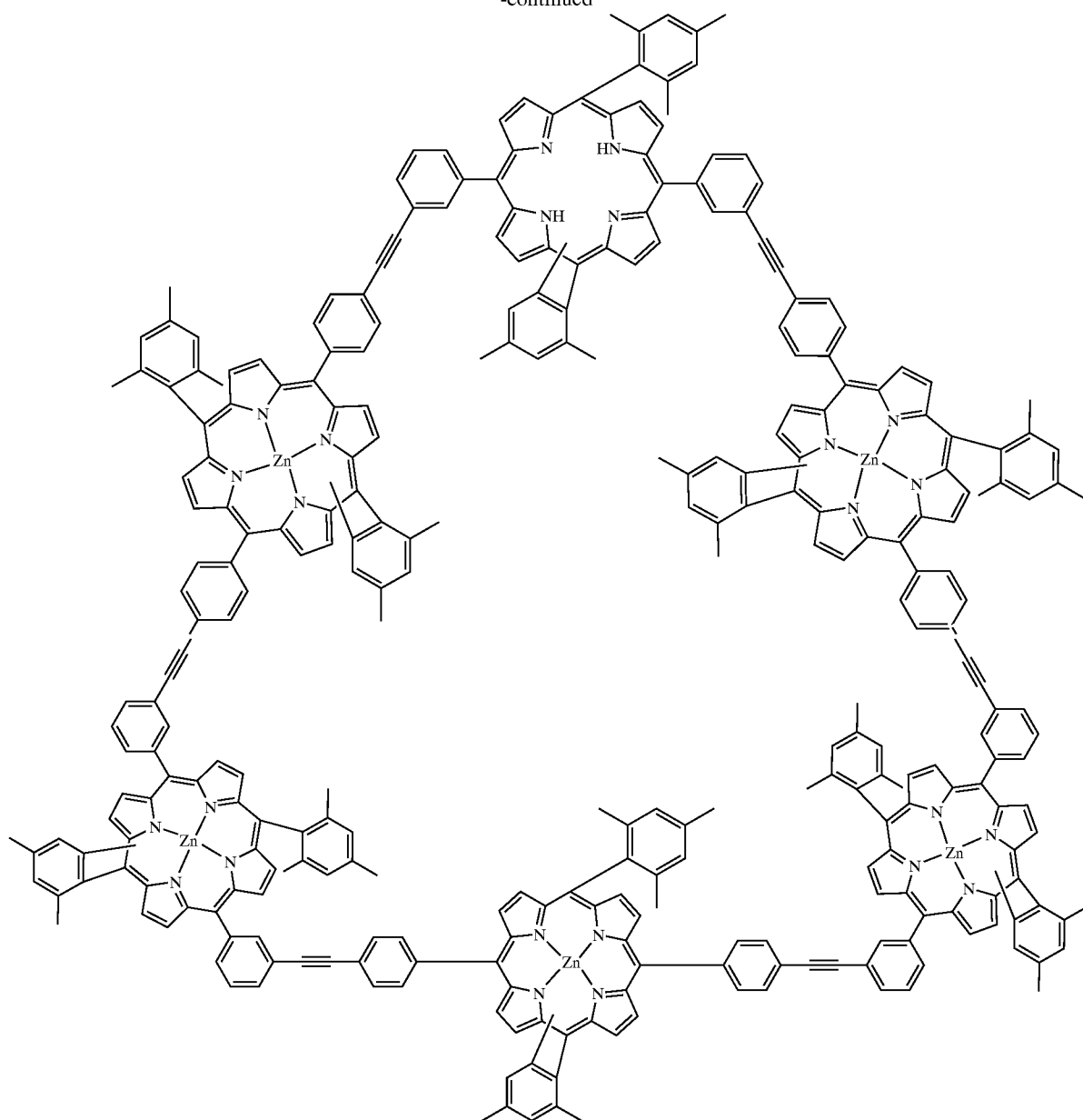
Cyclo-Zn 5 FbU
