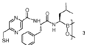
EC0501 Thio bortezomib
