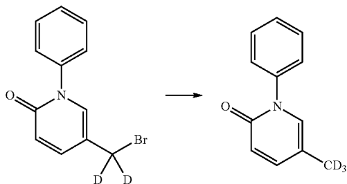
d 3 -5-(Methyl)-1-phenylpyridine-2(1H)-one
