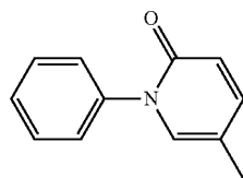
Pirfenidone
