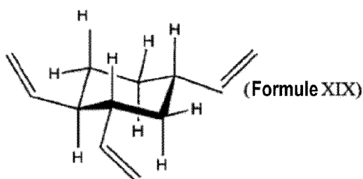
Isomère A
