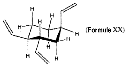
Isomère B
