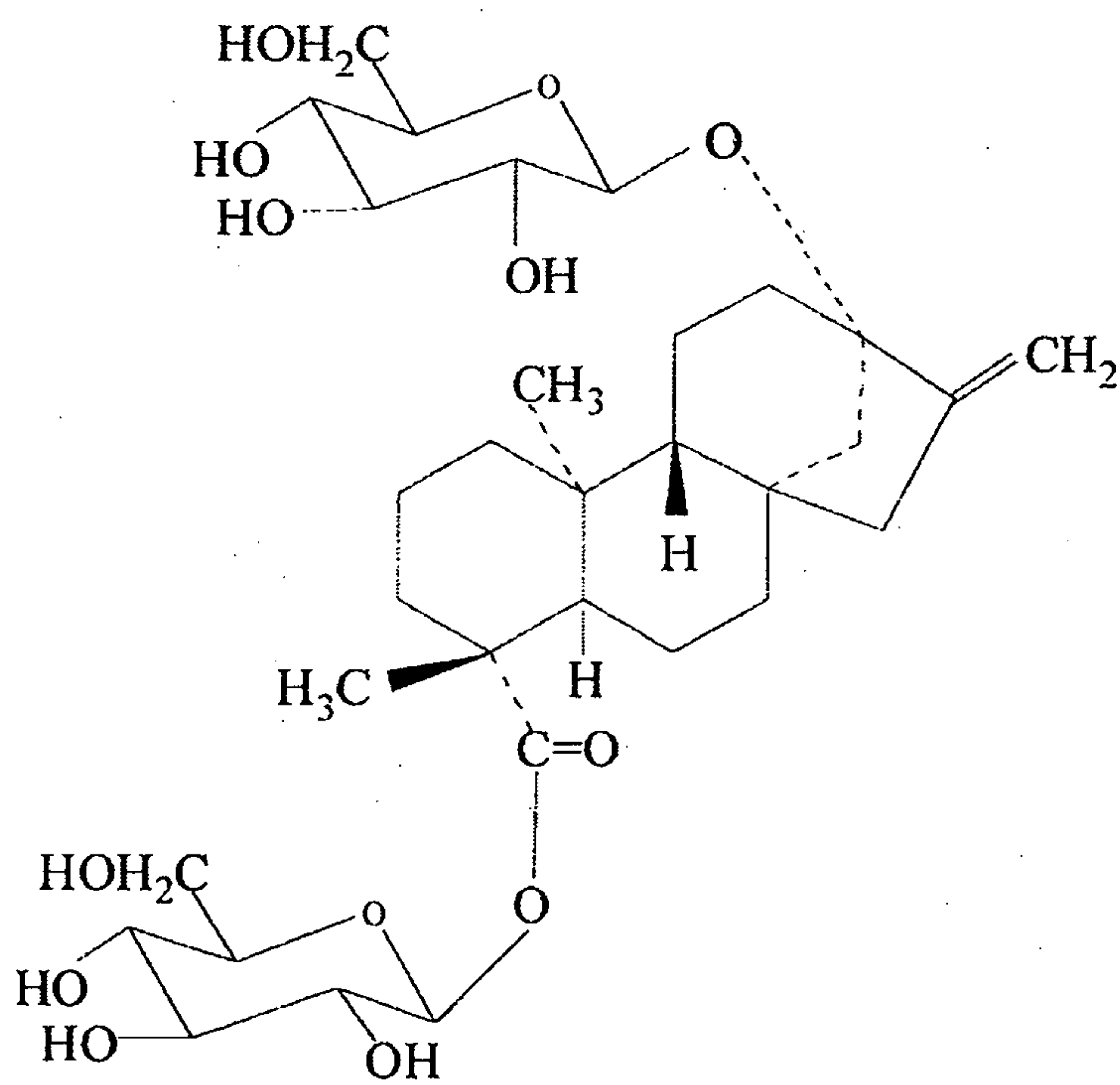
Rubusoside
