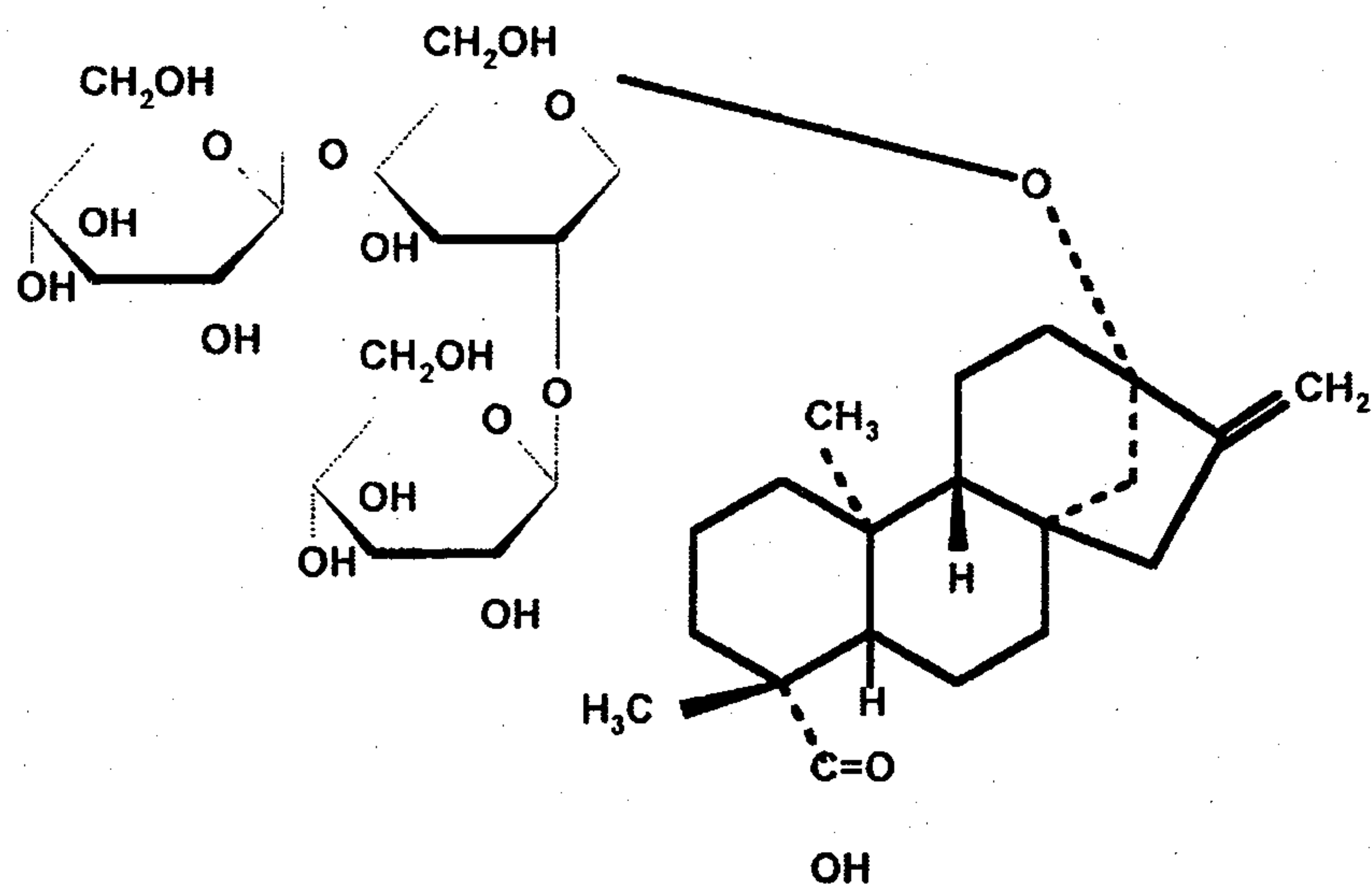
Rebaudioside B
