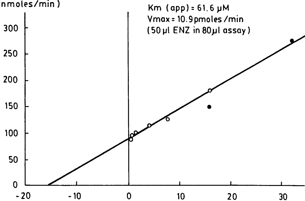
FIG.20 1/[ARG] (mM)
