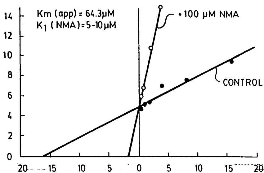
FIG.21 1/[ARG] (mM)
