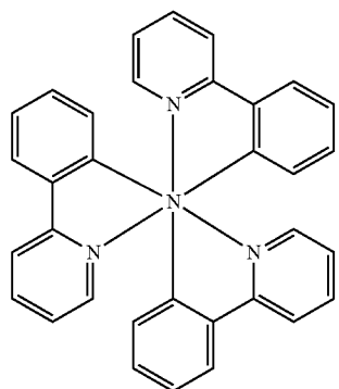
[Ir(ppy) 3 ]
