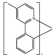
[Ir(mppy) 3 ]
