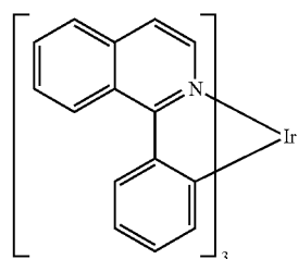
[Ir(piq) 3 ]
