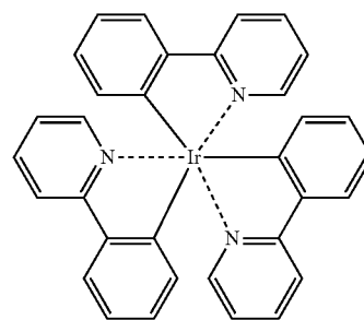
[Ir(ppy) 3 ]
