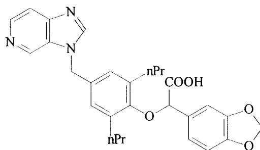
(L744453)
