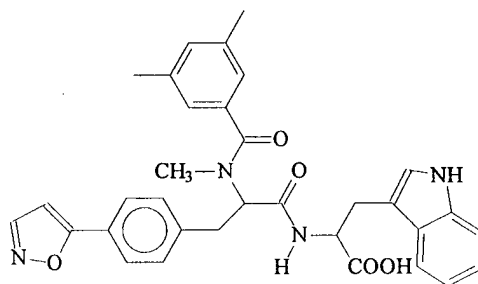
(IRL2796)
