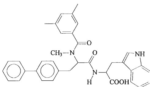
(IRL2500)
