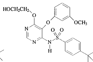
(Ro46-2005)
