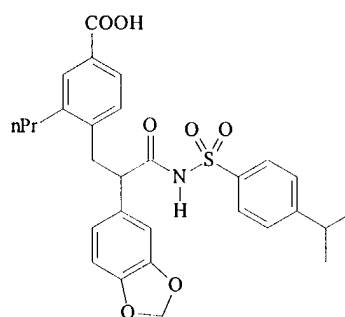
(L751281)
