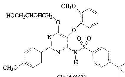
(Ro468443)
