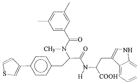
(IRL2500)
