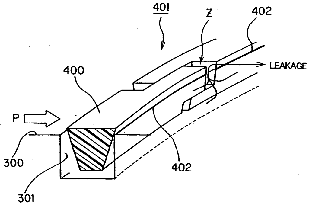
FIG. 38
