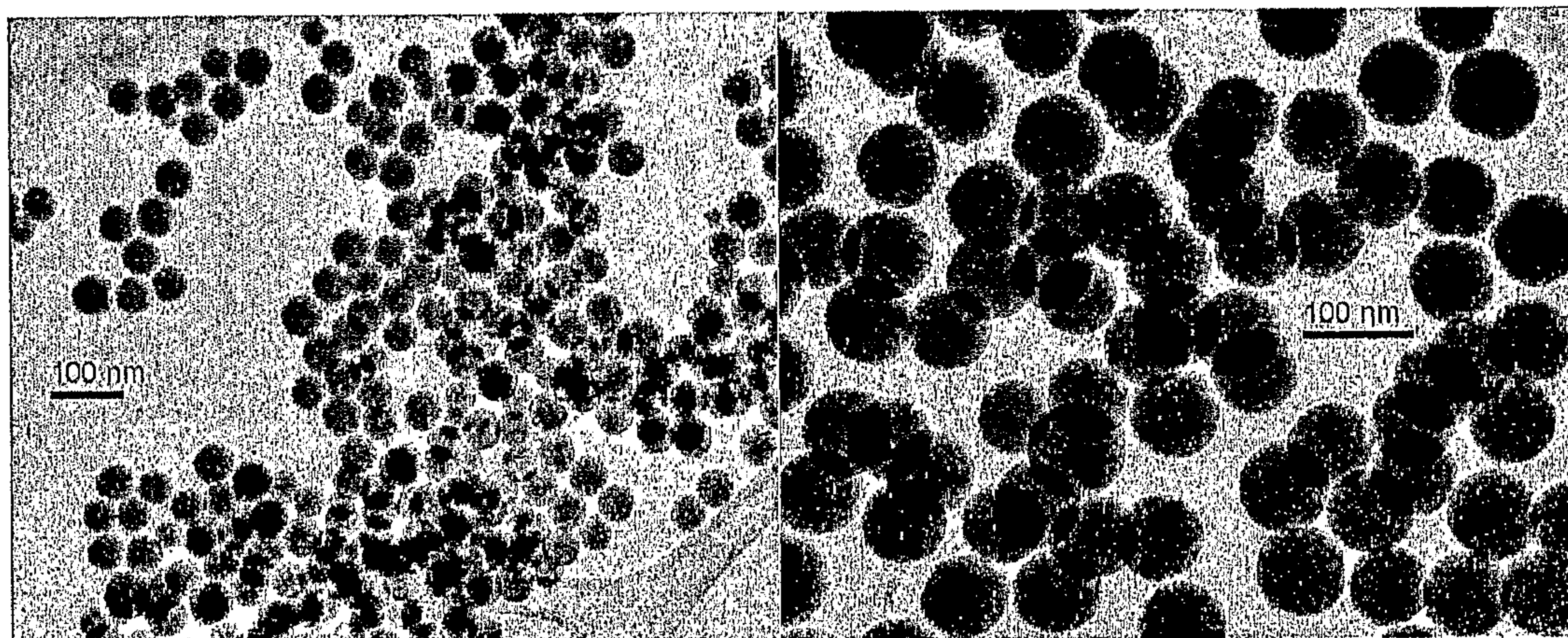
a: core (bar=100 nm)
