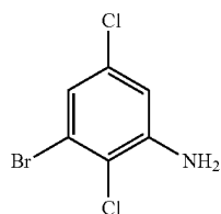
3-bromo-2,5-dichloroaniline
