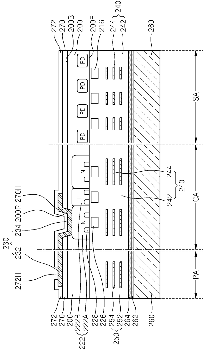
FIG. 8G
