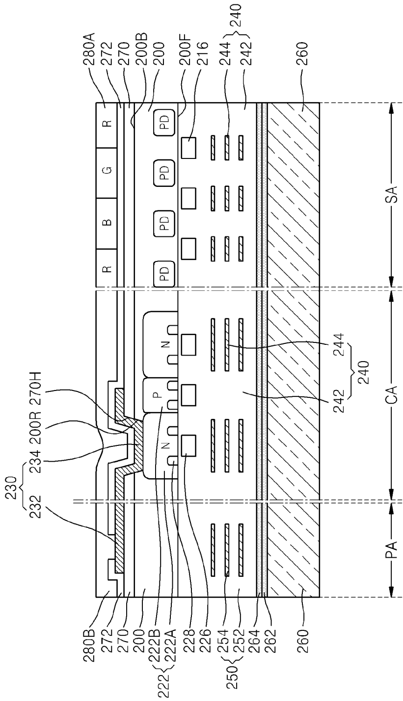
FIG. 8H
