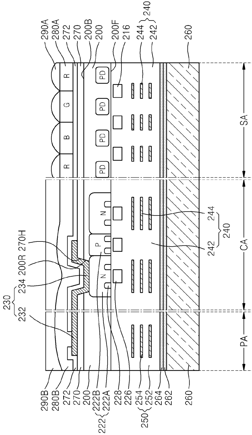
FIG. 8I
