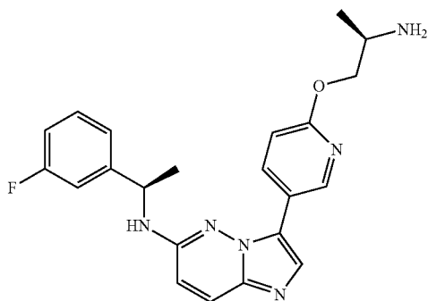
3-[6-[(2R)-2-Aminopropoxy]-3-pyridyl]-N-[(1R)-1-(3-fluorophenyl)ethyl]imidazo[1,2-b]pyridazin-6-amine
