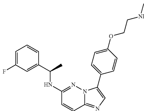
N-[(1R)-1-(3-Fluorophenyl)ethyl]-3-[4-(2-(methylamino)ethoxy)phenyl]imidazo[1,2-b]pyridazin-6-amine
