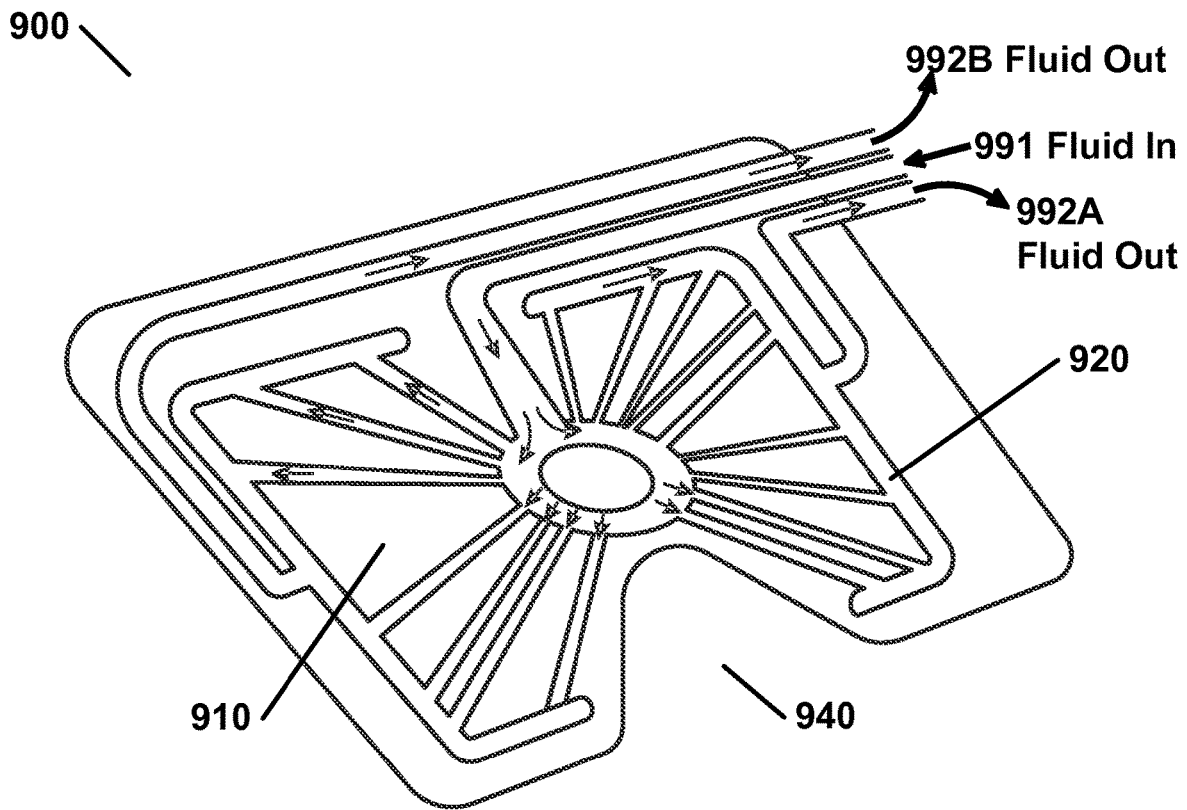
FIG. 9A
