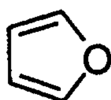
furan (furyl)
