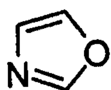
oxazole (oxazolyl)
