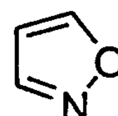
isoxazole (isoxazolyl)
