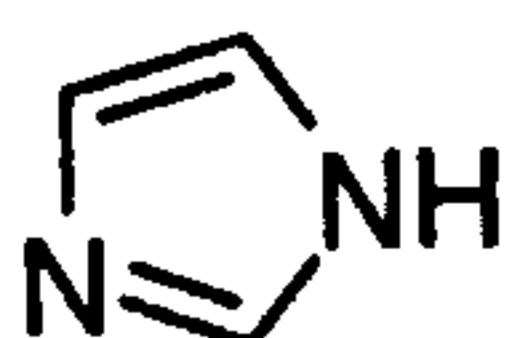
imidazole (imidazolyl)
