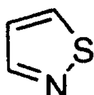
isothiazole (isothiazolyl)
