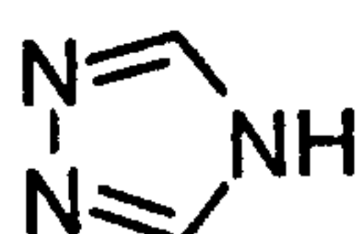
triazole (triazolyl)
