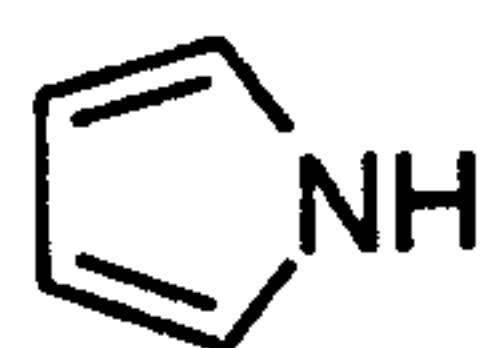
pyrrole (pyrrolyl)
