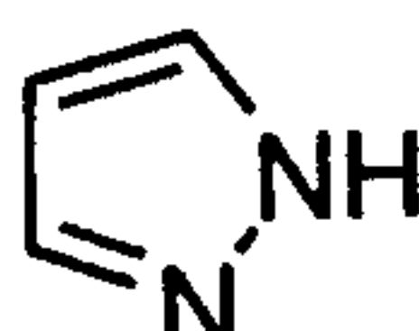
pyrazole (pyrazolyl)
