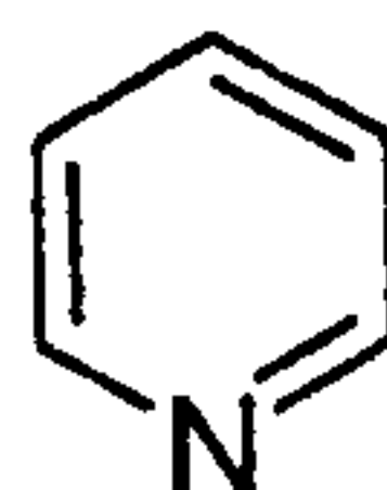
pyridine (pyridinyl)
