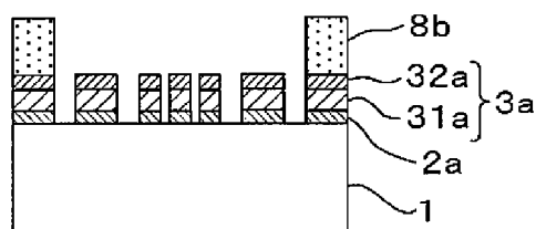
FIG. 5E
