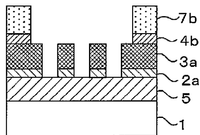
FIG. 4E
