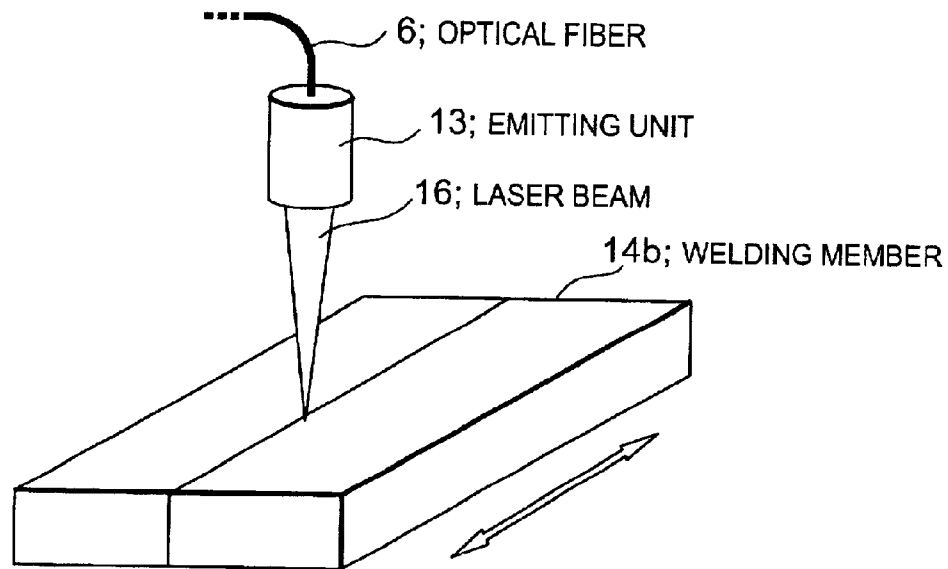
Fig.11(Prior Art)
