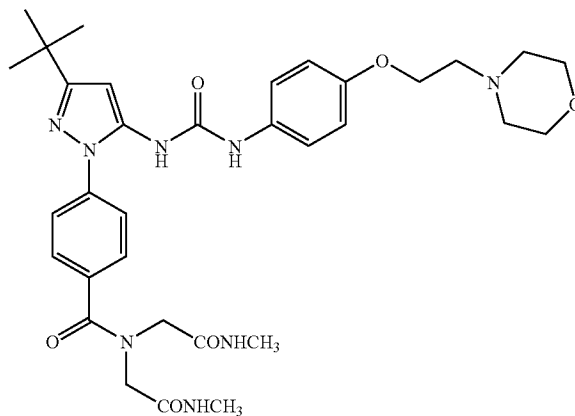
Example 129
