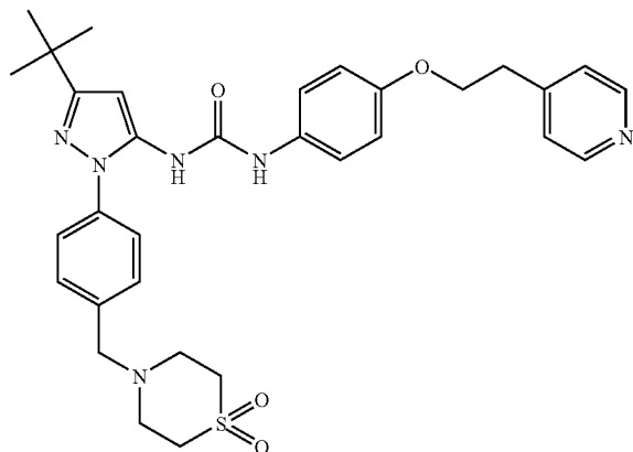
Example 119
