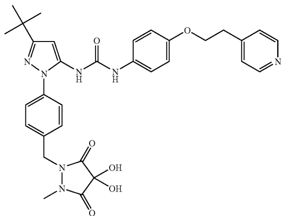
Example 107
