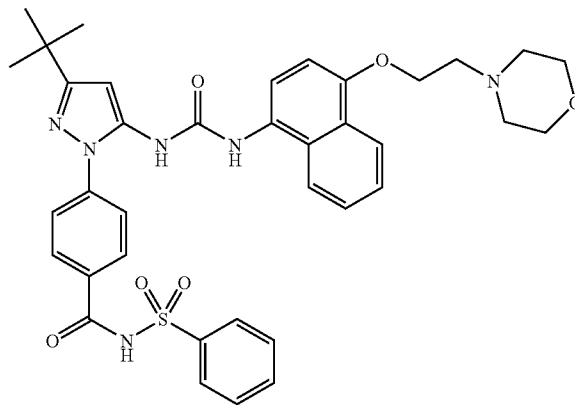
Example 122
