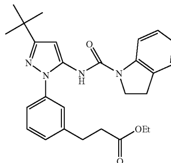
Example 176
