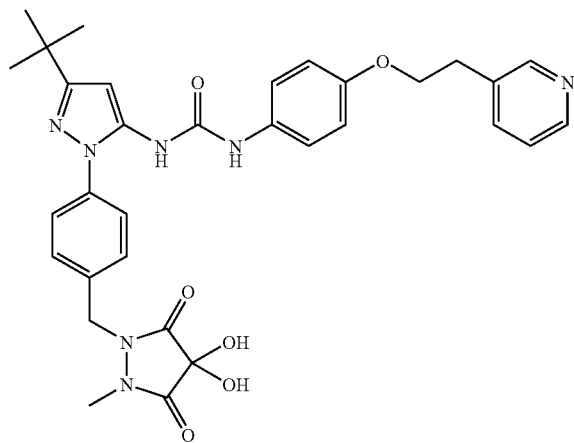
Example 108
