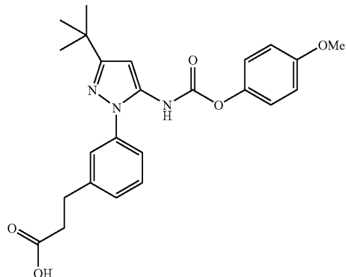
Example 171
