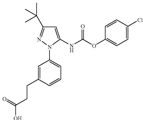
Example 169
