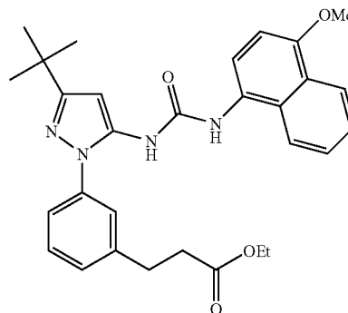
Example 174
