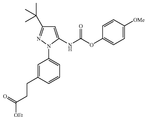
Example 170
