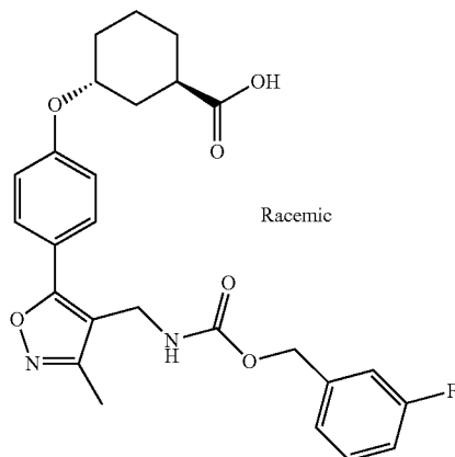
(±)-Trans-3-(4-(4-(((3-fluoro-benzyl)oxy)carbonyl)amino)methyl)-3-methylisoxazol-5-yl)phenoxy)cyclohexanecarboxylic acid
