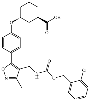
(±)-Trans-3-(4-(4-(((2-chloro-benzyl)oxy)carbonyl)amino)methyl)-3-methylisoxazol-5-yl)phenoxy)cyclohexanecarboxylic acid
