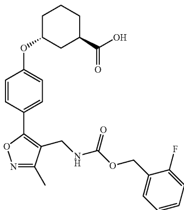
(±)-Trans-3-(4-(4-(((2-fluorobenzyl)oxy)carbonyl)amino)methyl)-3-methylisoxazol-5-yl)phenoxy)cyclohexanecarboxylic acid
