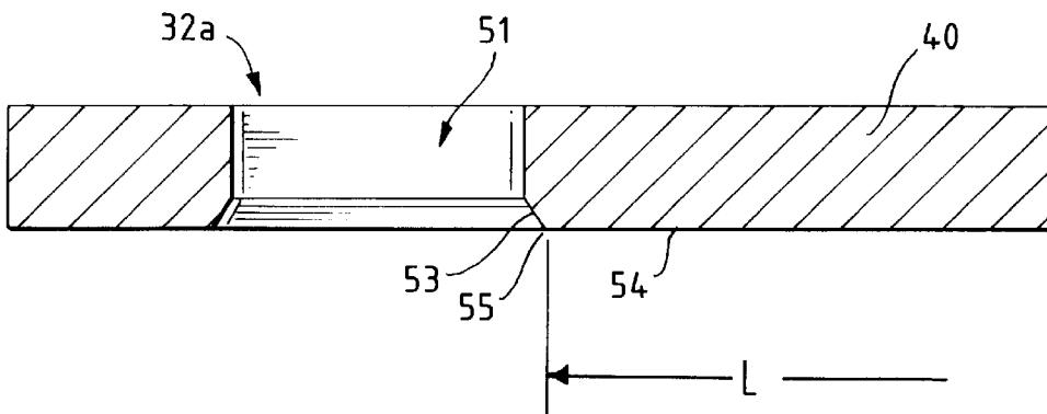
FIG. 4B SECTION A-A
